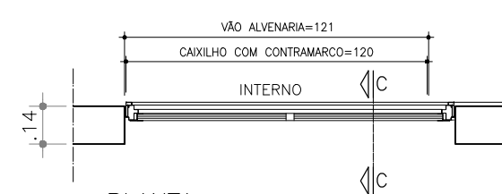
PLANTA JANELA MAXIMAR 1,20X0,80 BRINQUEDOTECA/SALAS DE ATENDIMENTO ESC 1:25
