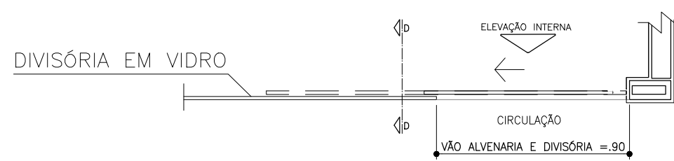
PLANTA ESCALA 1:25 PVO1 – PORTA DE VIDRO/INTERNA C/ FERRAGEM E FECHADURA ESPAÇO CULINÁRIO – 1 UNIDADE
