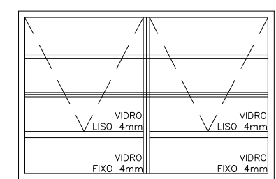
VISTA EXTERNA ESCALA 1:25
