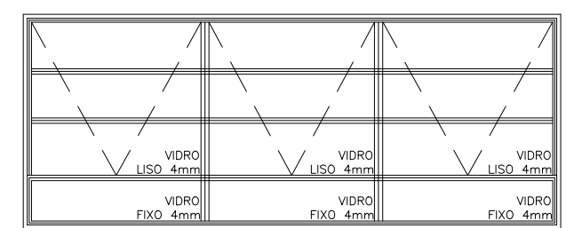
VISTA EXTERNA ESCALA 1:25
