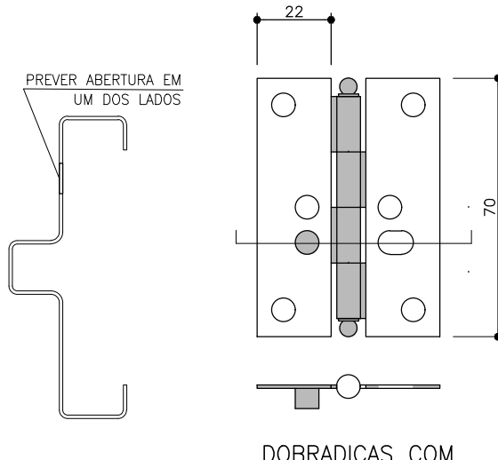
DOBRADIÇAS COM TRAVA DE SEGURANÇA ESCALA 1:2
