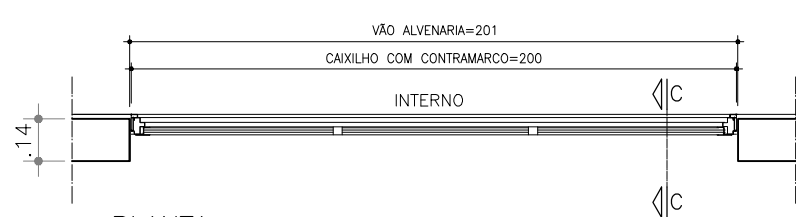
PLANTA JANELA MAXIMAR 2,00X0,80 ESPAÇO CULINÁRIO ESC 1:25
