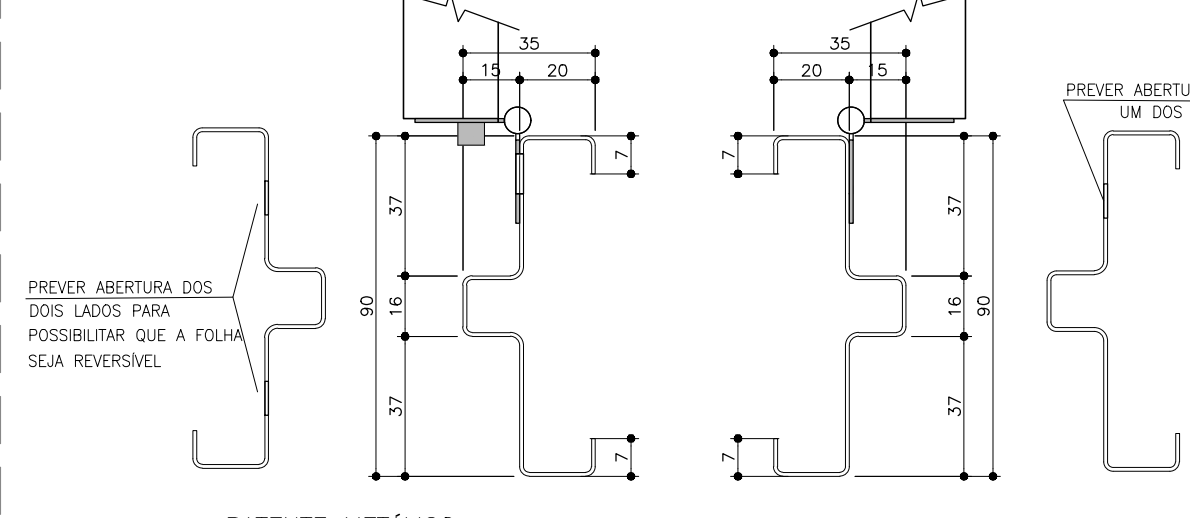
BATENTE METÁLICO COM 2 REBAIXOS DETALHE TÍPICO ESCALA 1:2 * MEDIDAS EM MILÍMETROS DETALHE BATENTE KIT PORTA ESC.: 1:2
