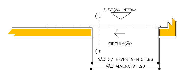
PLANTA ESCALA 1:25 PVO2 – PORTA DE VIDRO/INTERNA C/ FERRAGEM E FECHADURA ESPAÇO BRINQUEDOTECA – 1 UNIDADE
