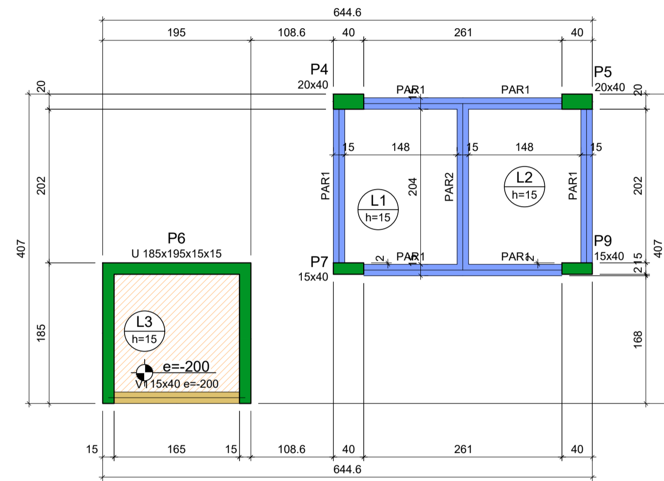
FORMAS RESERVATÓRIO - NÍVEL 1497cm ESC.: 1/50
