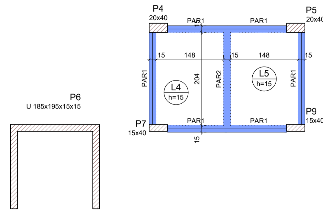
FORMAS RESERVATÓRIO - NÍVEL 1287cm ESC.: 1/50
