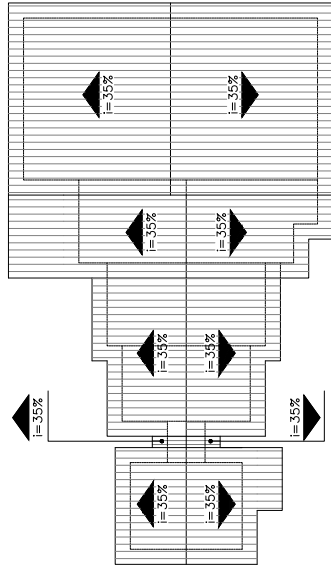
COBERTURA 1:50
