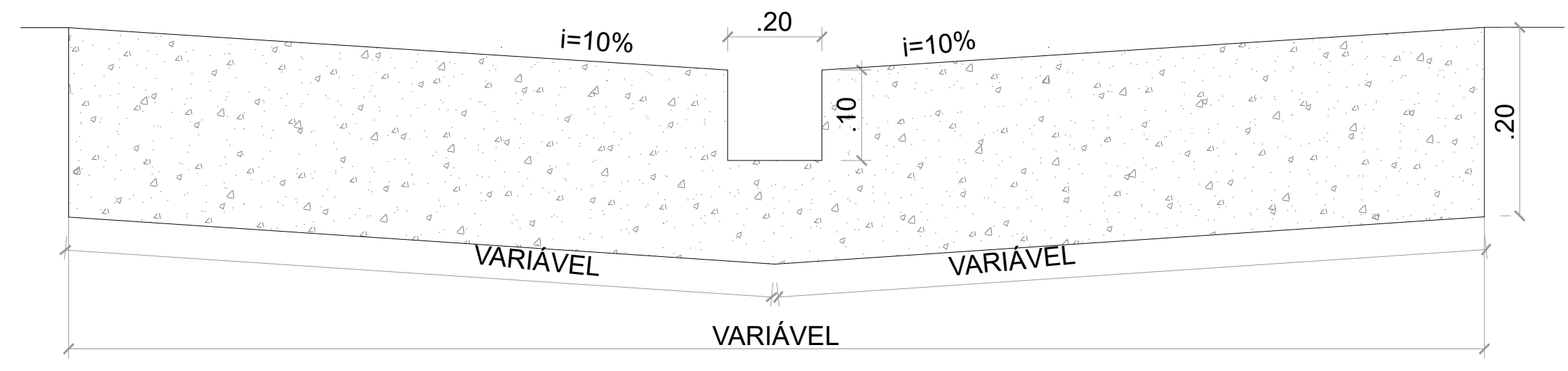
DETALHE SARJETÃO SEM ESCALA
