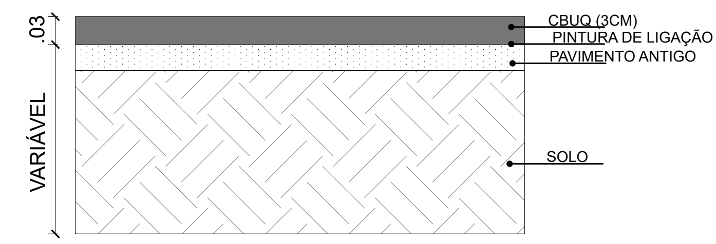
ESTRUTURA PAVIMENTO SEM ESCALA
