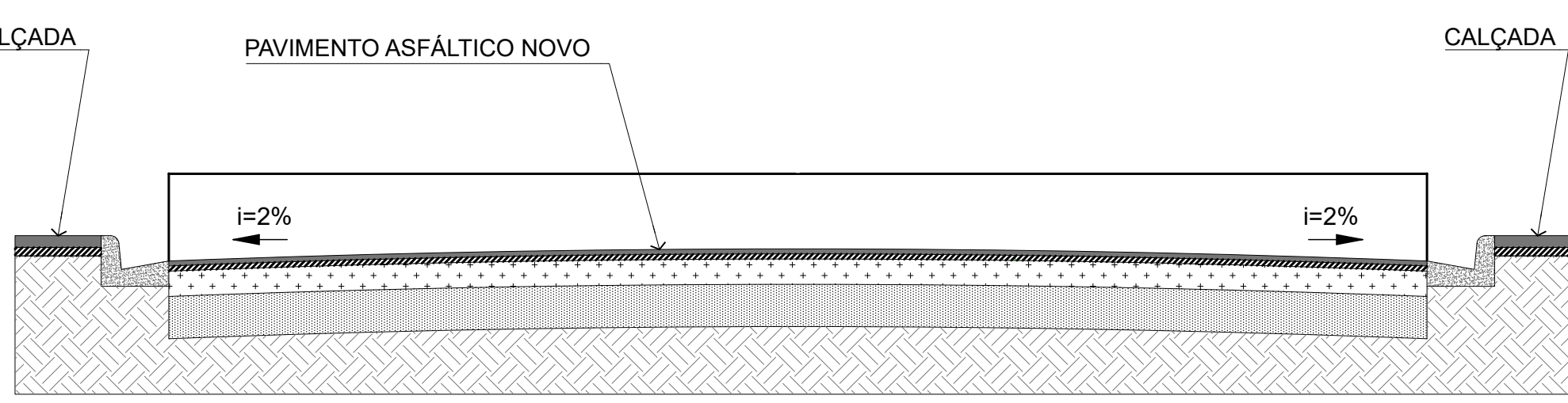
PERFIL TÍPICO DA PAVIMENTAÇÃO SEM ESCALA
