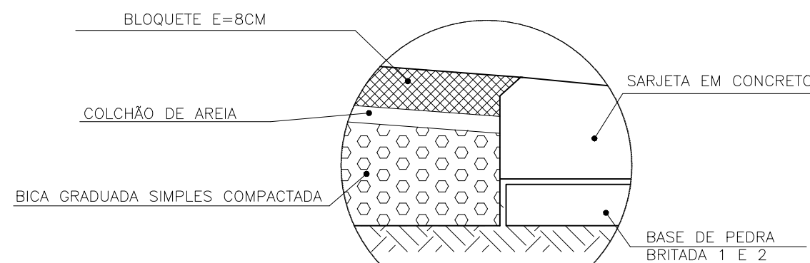
DETALHE A S/ESCALA
