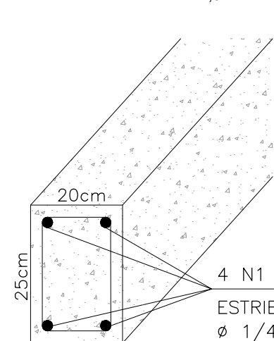
VIGA DE TRAVAMENTO S/ ESC.
