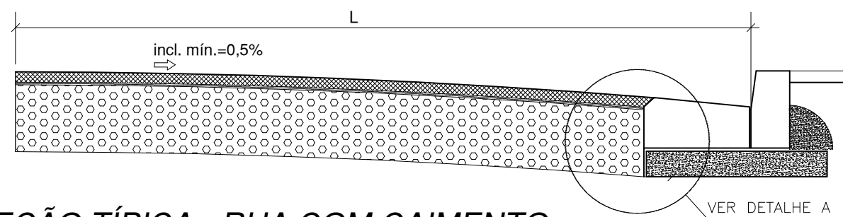
SEÇÃO TÍPICA - RUA COM CAIMENTO S/ ESCALA
