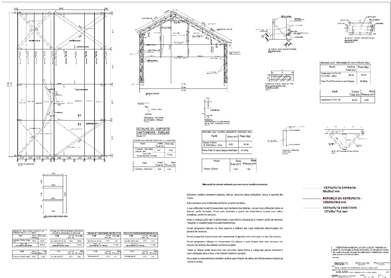
Foto 04- Projeto Metálica fl. 01
