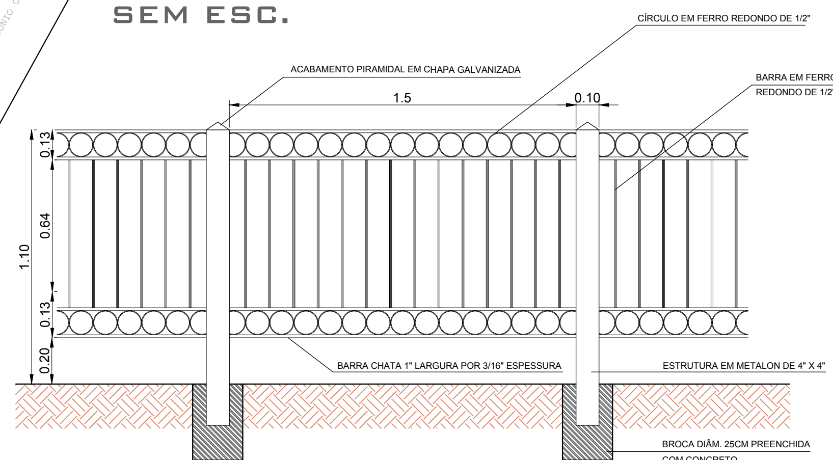
DETALHAMENTO GRADIL SEM ESC.
