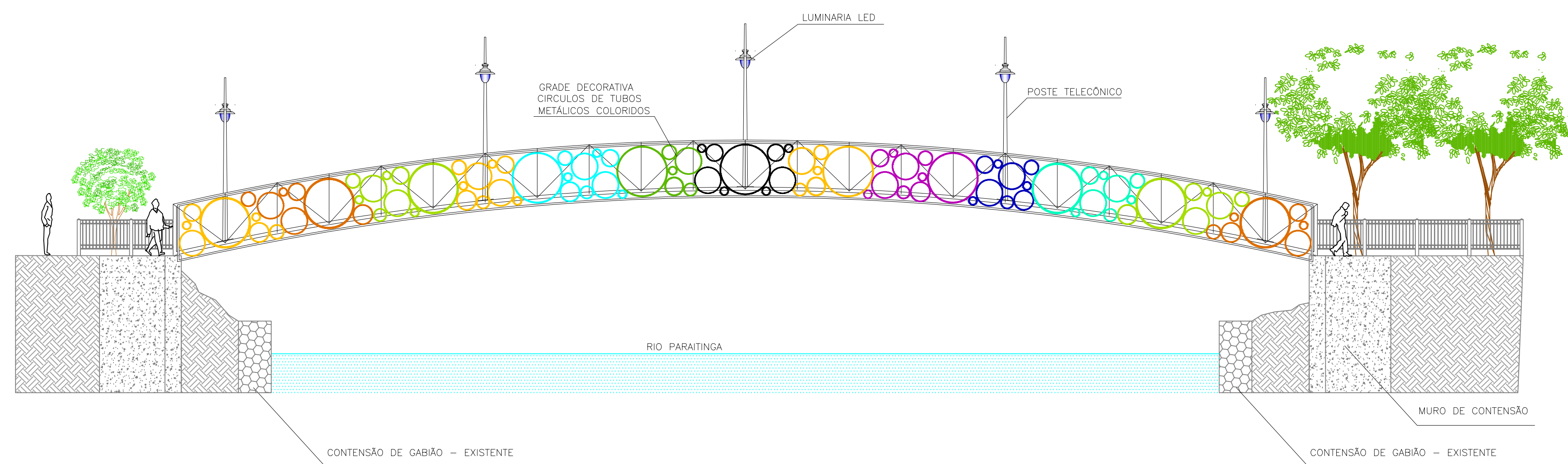
ELEVAÇÃO ESC. 1:100
