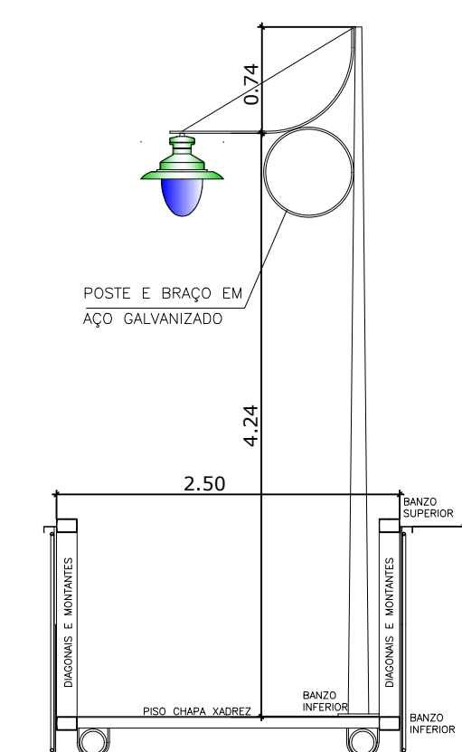
CORTE TRANSVERSAL ESC. 1:50
