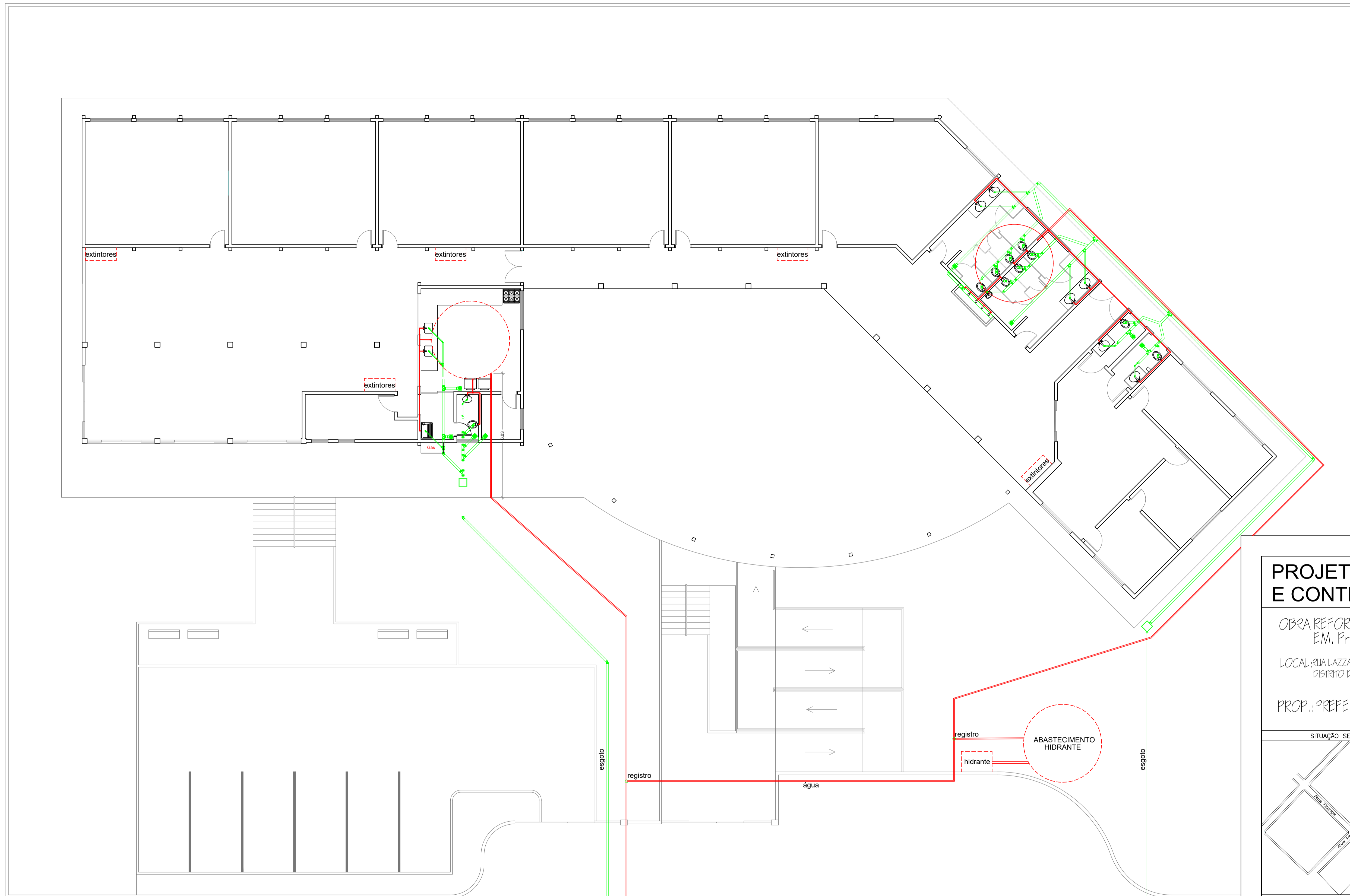
PLANTA - PROJETO HIDRÁULICO ESC. 1/100
