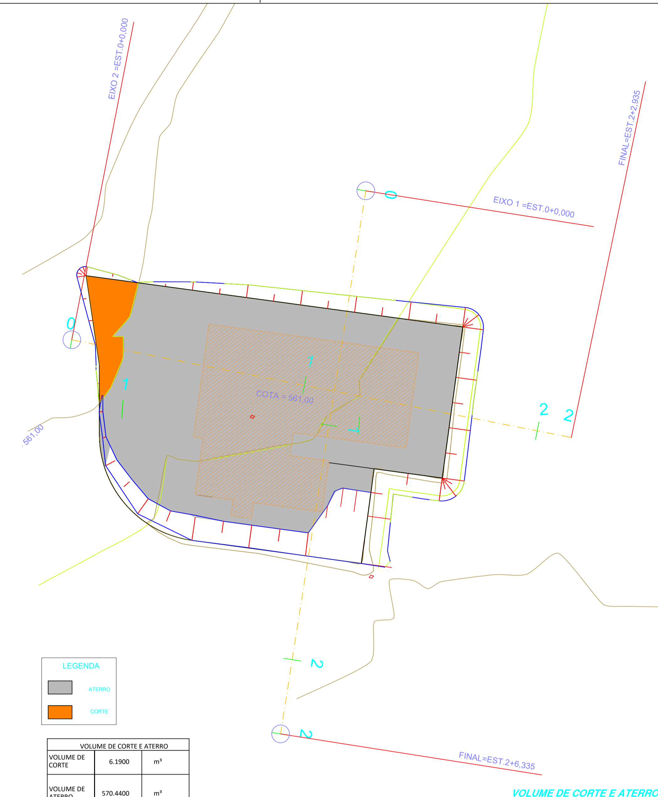
VOLUME DE CORTE E ATERRO Escala 1:200
