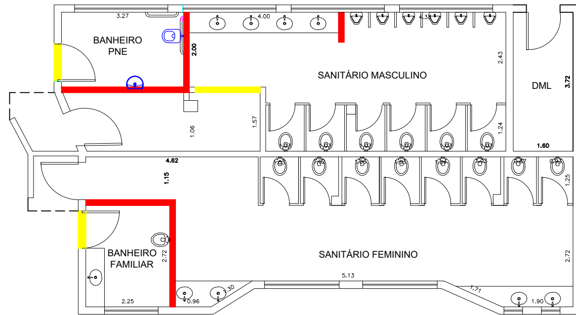
PROJETO DE REFORMA E ADEQUAÇÃO ESC 1:100
