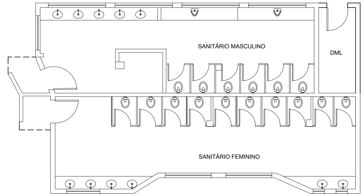
LAYOUT ATUAL ESC 1:100
