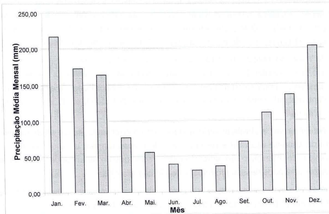
Figura 4: Precipitação Média Mensal (mm).
