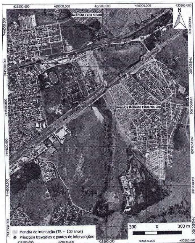
Figura 8: Principais travessias e pontos de intervenções no Ribeirão dos Mudos. Fonte: Plano Diretor de Macrodrenagem do Município de Caçapava (2017).
