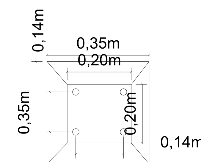
DETALHE 3 Sem Escala
