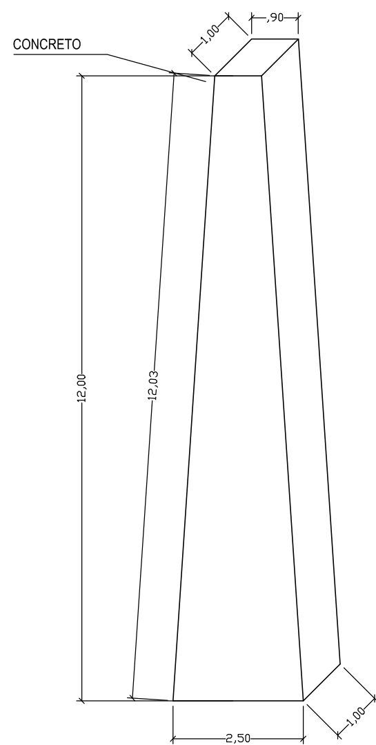
DETALHE ESTRUTURA CONCRETO ESC: 1/100
