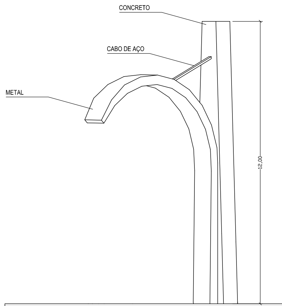
PERSPECTIVA ESC: 1/100
