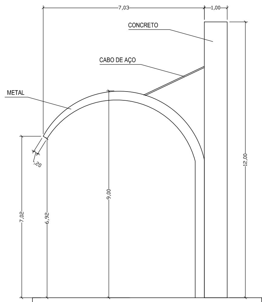
CORTE ESC: 1/100
