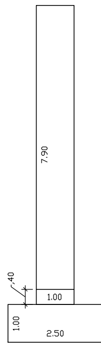
PLANTA TOTTEN - LETREIRO ESC: 1/100
