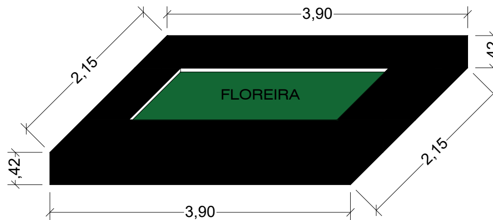
DETALHE DO BANCO DE MADEIRA E ALVENARIA ESC 1:50
