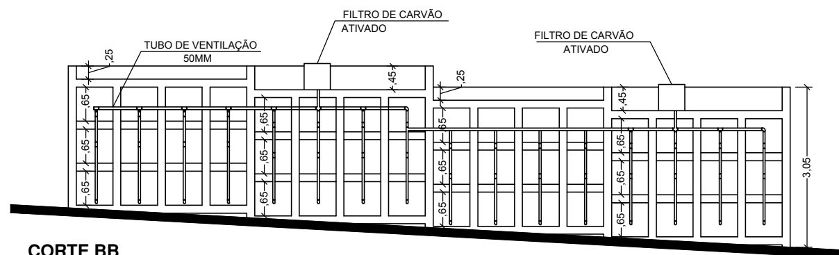
CORTE BB
