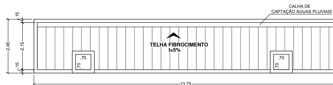
PLANTA DE COBERTURA GAVETÁRIO ESC: 1/100
