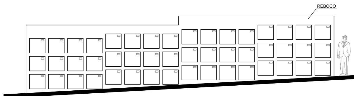
FACHADA FRONTAL ESC: 1/100
