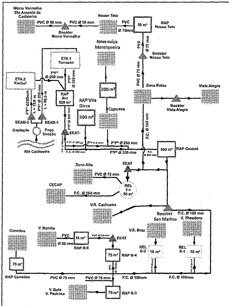
Figura 2 – Esquema do Sistema de Abastecimento de Água do município
