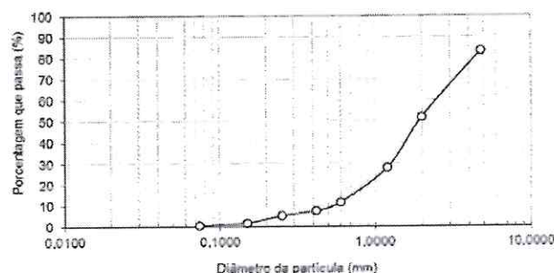
Figura 2 - Curva granulométrica da borracha utilizada. Fonte: Própria.
