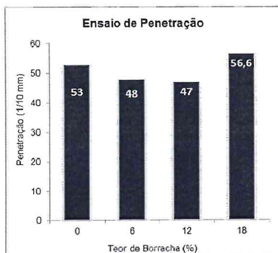
Figura 4 - Resultados Ensaio de Penetração. Fonte: Própria.
