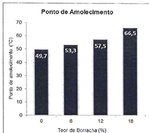
Figura 5 - Resultado do ensaio de Ponto de Amolecimento.
