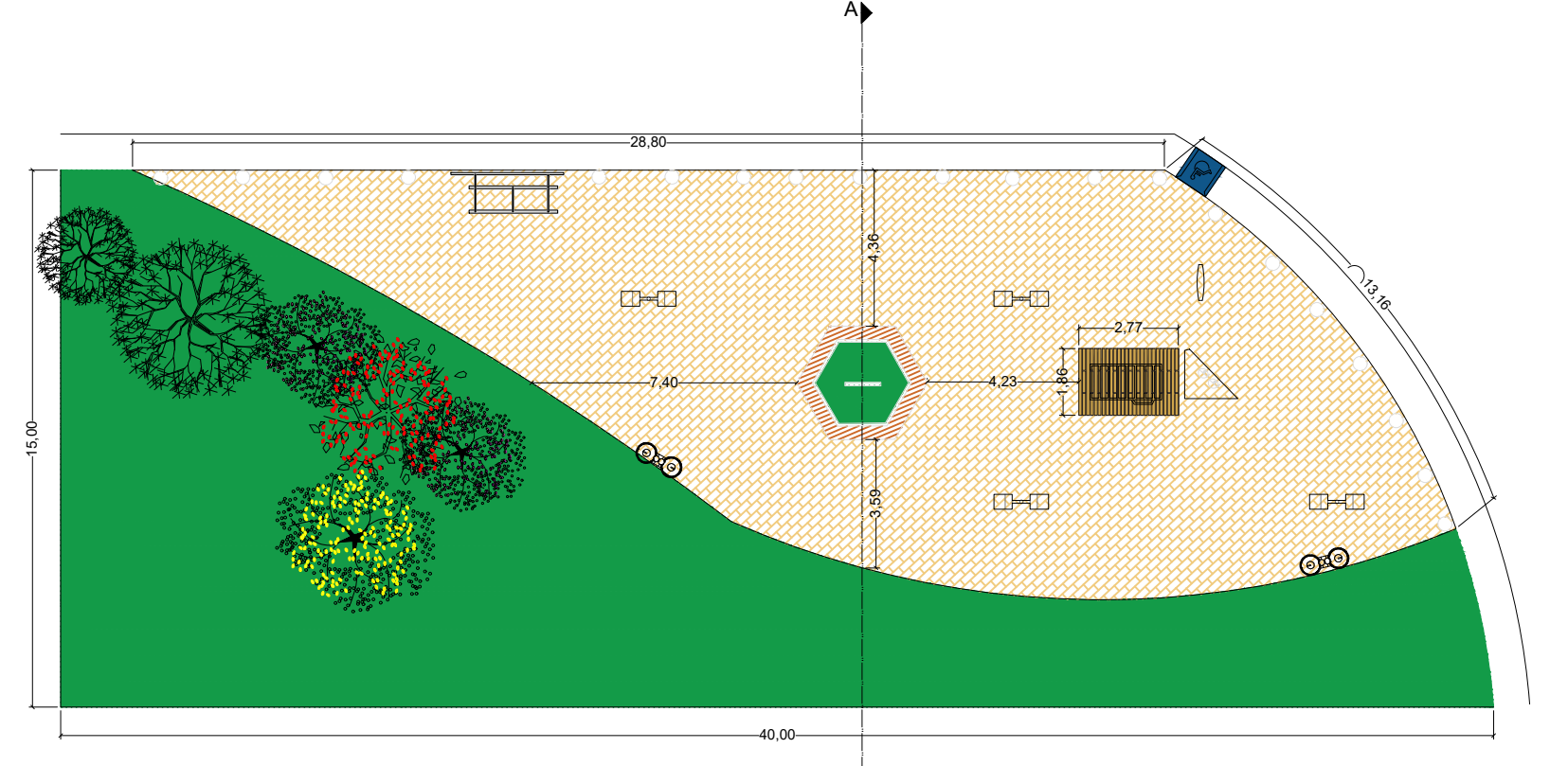
3 PLANTA PONTO 2 ESC: 1/200
