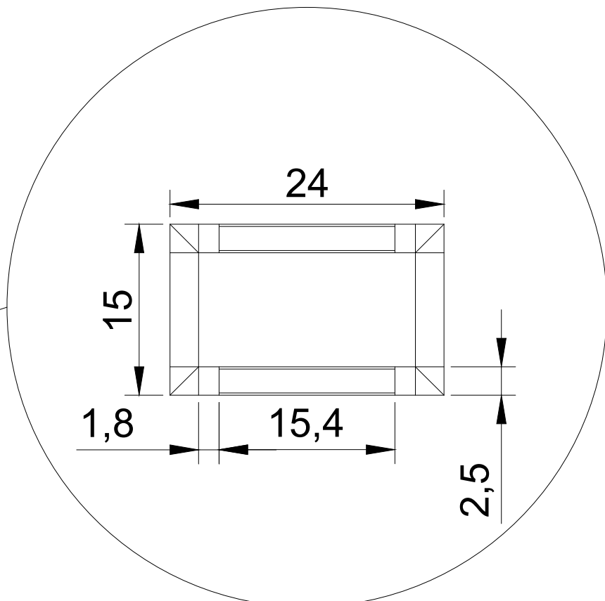
6 DETALHE TAXÃO S/ ESCALA
