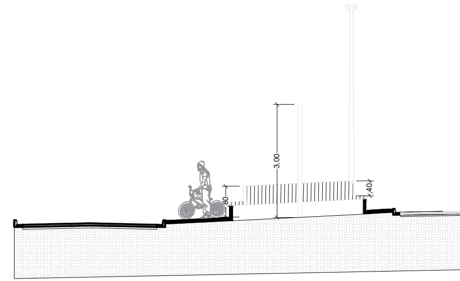
4 CORTE AA PONTO 1 ESC: 1/100
