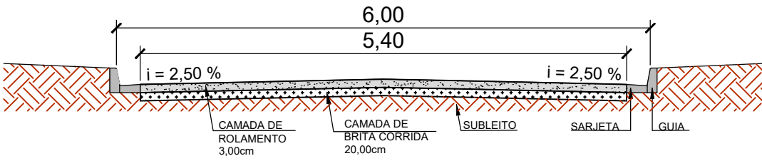
SECÇÃO TRANSVERSAL MÉDIA S/ ESC.
