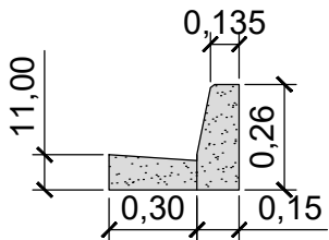
SARJETA E MEIO FIO S/ ESC.
