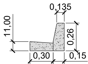
SARJETA E MEIO FIO S/ ESC.
