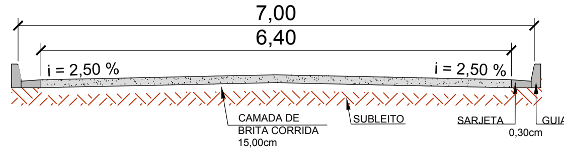
SECÇÃO TRANSVERSAL MÉDIA - Trecho das demais Ruas S/ ESC.
