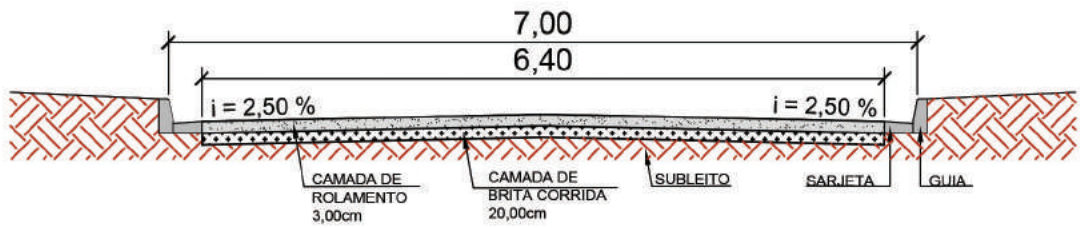
SECÇÃO TRANSVERSAL MÉDIA - AVENIDA B S/ ESC.
