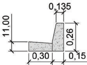
SARJETA E MEIO FIO S/ ESC.
