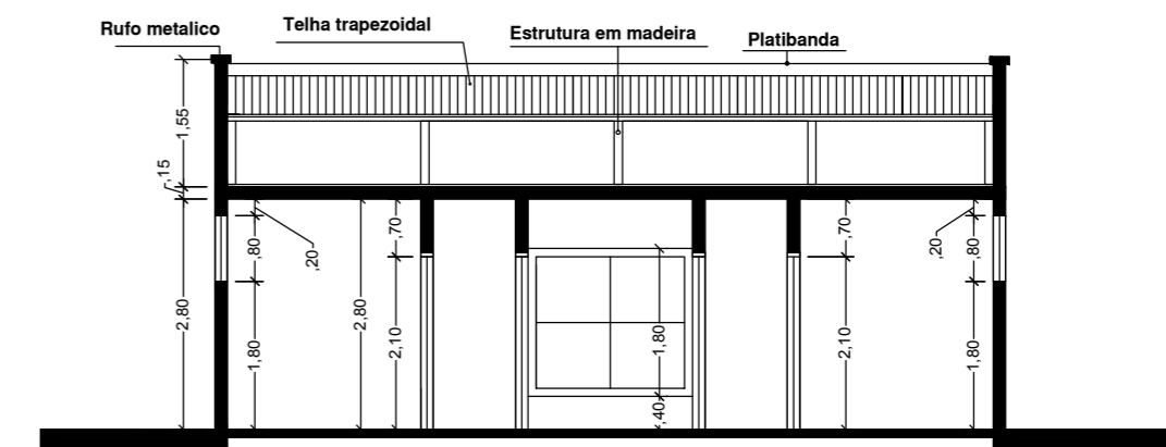
CORTE ESQUEMÁTICO AA ESC 1:100
