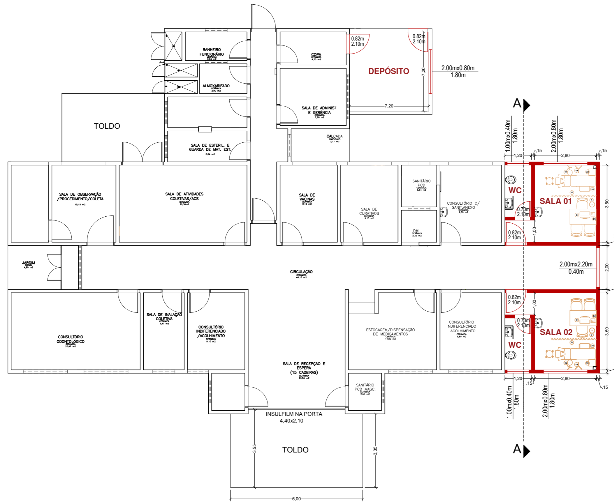
PLANTA: AMPLIAÇÃO DA UBS BATATUBA ESC 1:100
