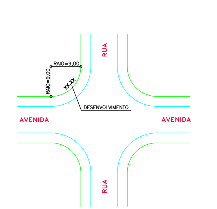
DETALHE DO CRUZAMENTO DAS VIAS (SEM ESCALA)
