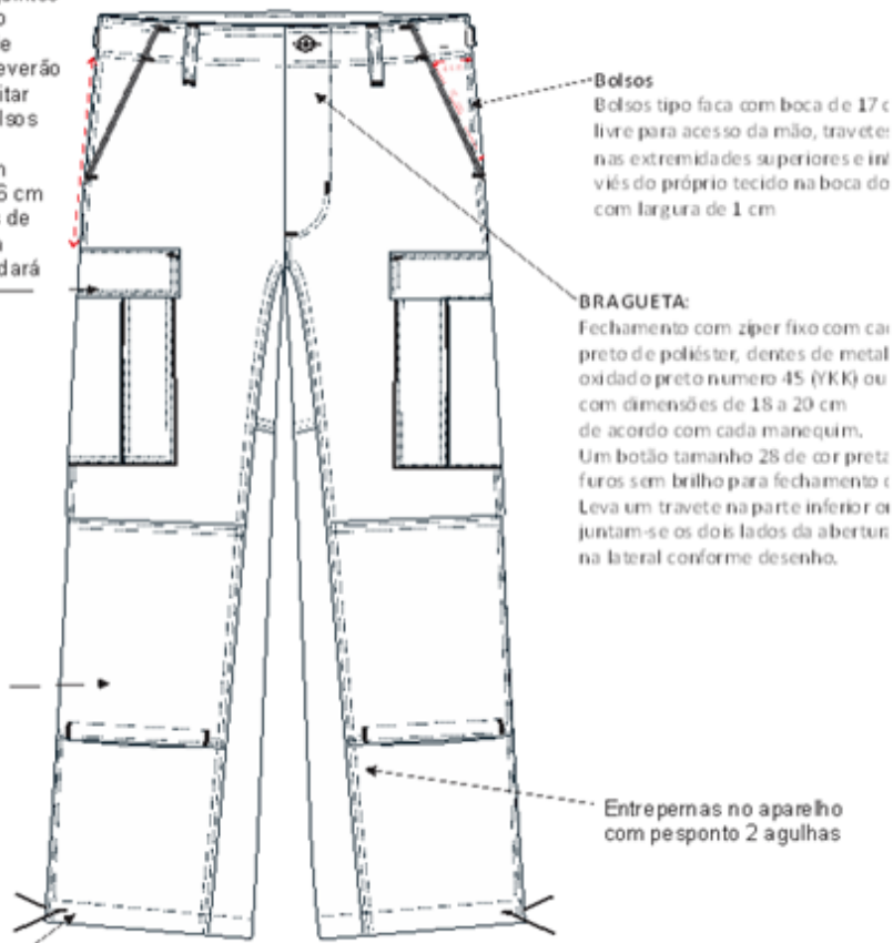
Figura 8: Visão Frontal da Calça Tática
