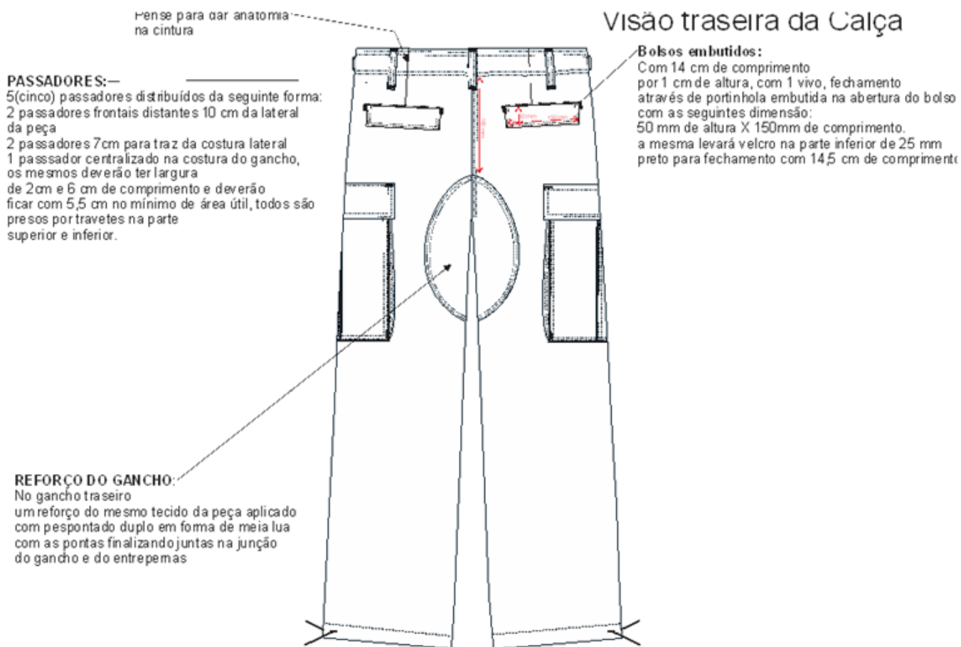
Figura 9: Visão Traseira da Calça Tática
