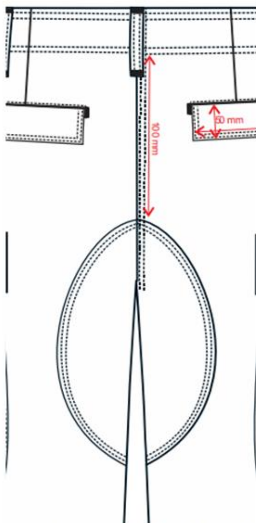
Figura 7: Características da Calça Tática
