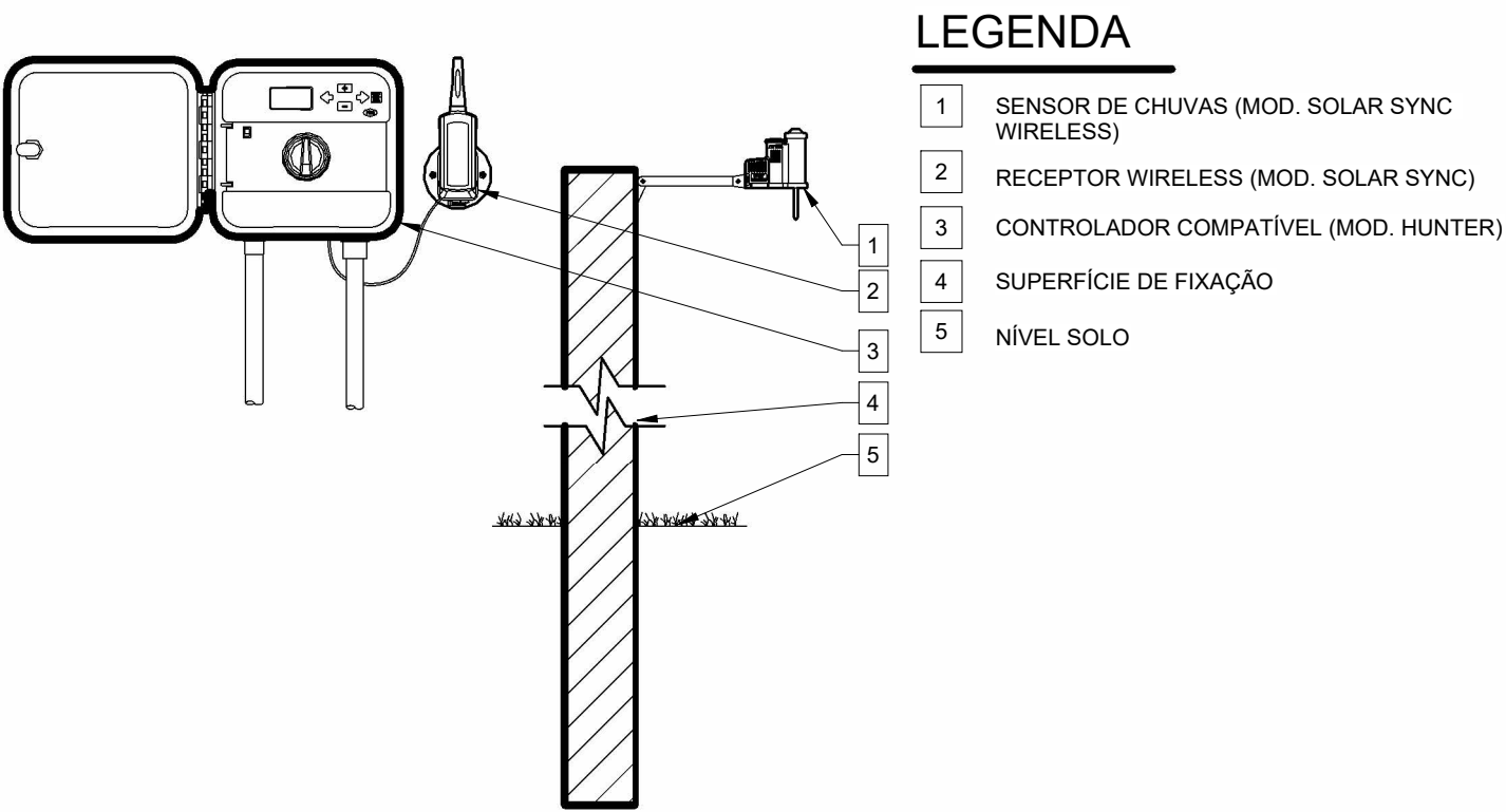
DETALHE DE SENSOR DE CHUVA (MOD. HUNTER SOLAR SYNC WIRELESS S.SS.04 COM CONTROLE REMOTO DE PAREDE)
