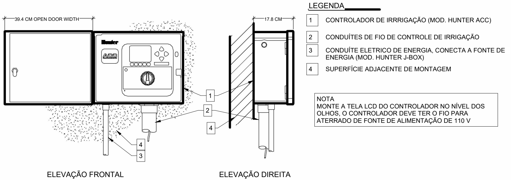
DETALHE DE INSTALAÇÃO DE PAREDE DO CONTROLADOR (MOD. HUNTER C.ACC.01 ACC)
