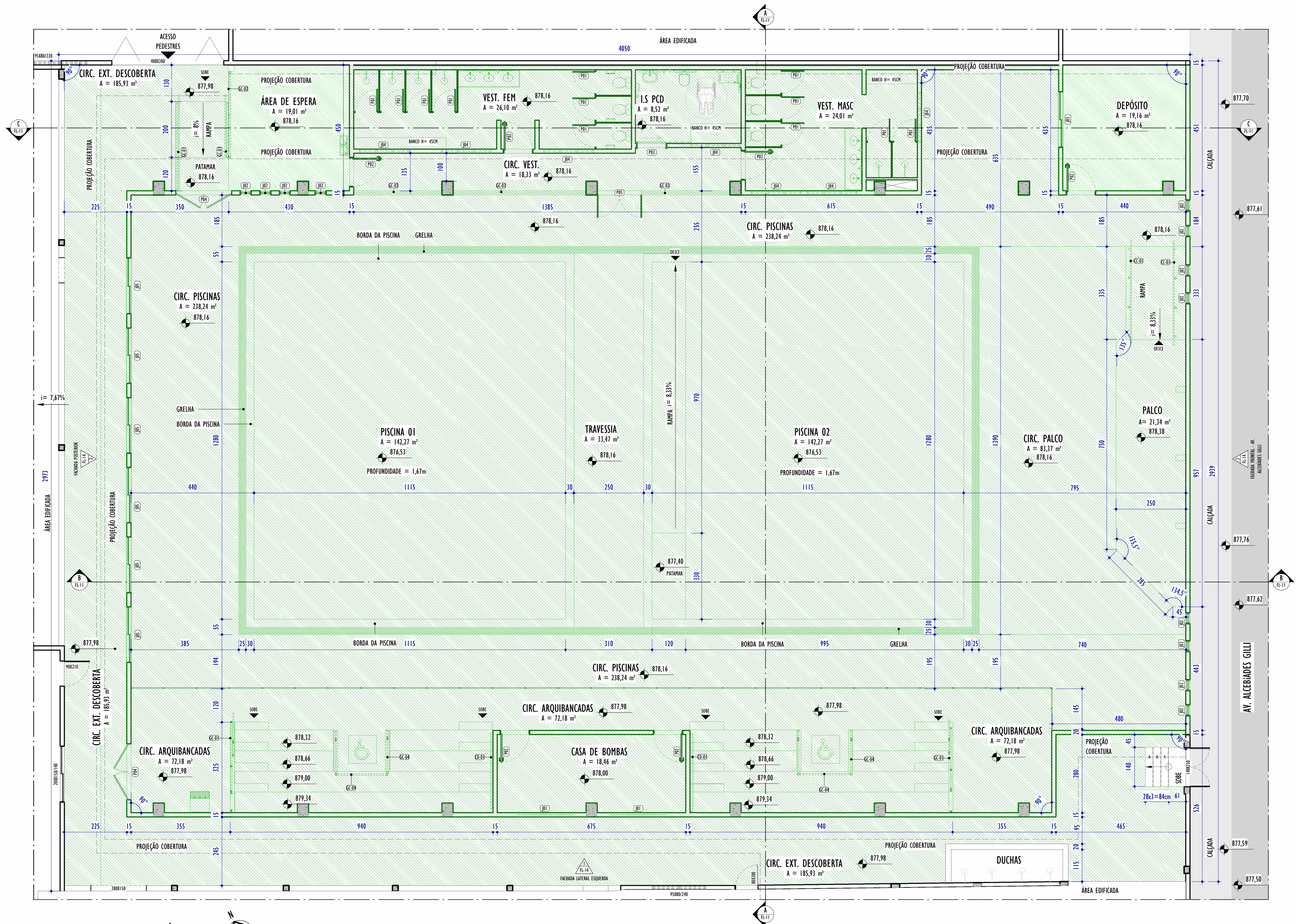
REFORMA - PLANTA TÉRREO ESCALA: 1 : 75
