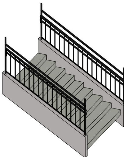
Figura 27 - Guarda Corpo com Corrimão Duplo – 1 Lado
