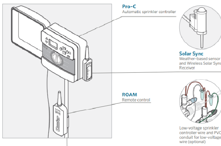
Figura 45 - Instalação do Controlador
