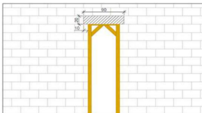
Figura 6 – Detalhe ilustrativo de vergas de portas.
