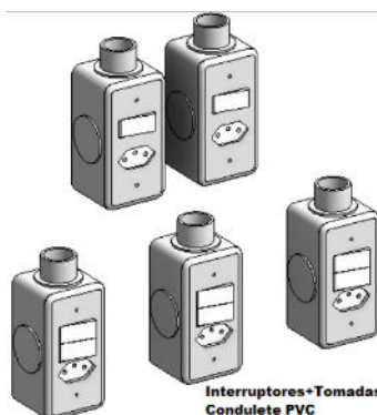
Figura 51 - Interruptores + Tomadas em Conduletes de PVC
