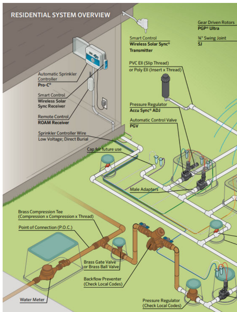
Figura 36 - Exemplo de sistema de irrigação de pequeno porte.
