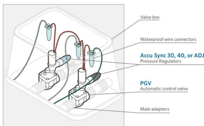
Figura 46 - Ligação das Válvulas Solenoides
