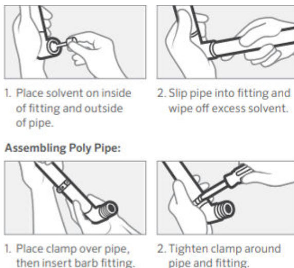
Figura 40 - Procedimento de colagem e instalação das conexões da linha de distribuição.
