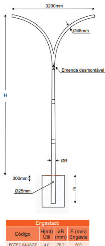
Figura 54 - Poste Telecônico Curvo Duplo - Dimensões
