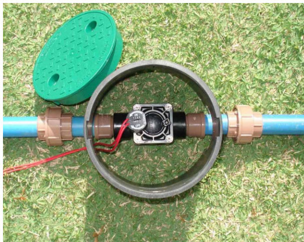
Figura 42 - Instalação de Válvulas
