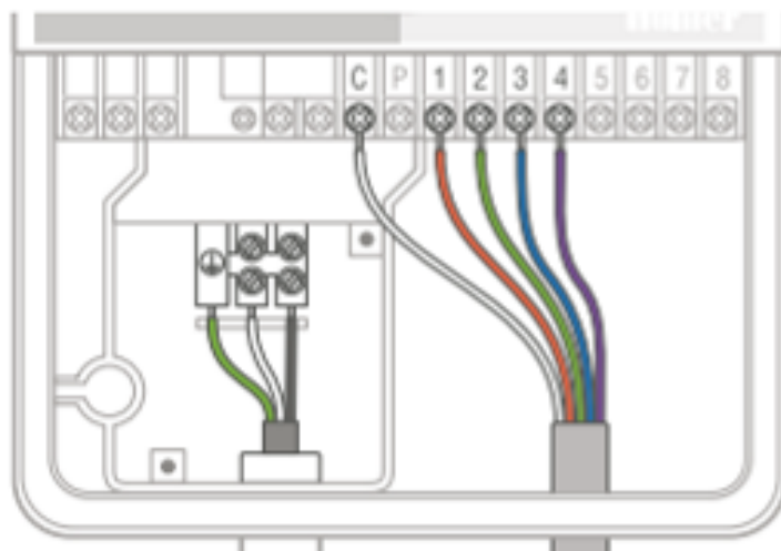
Figura 44 - Use fio de irrigação com código de cores para conectar as válvulas ao controlador. Você precisará de um fio para cada válvula, mais um fio comum.
