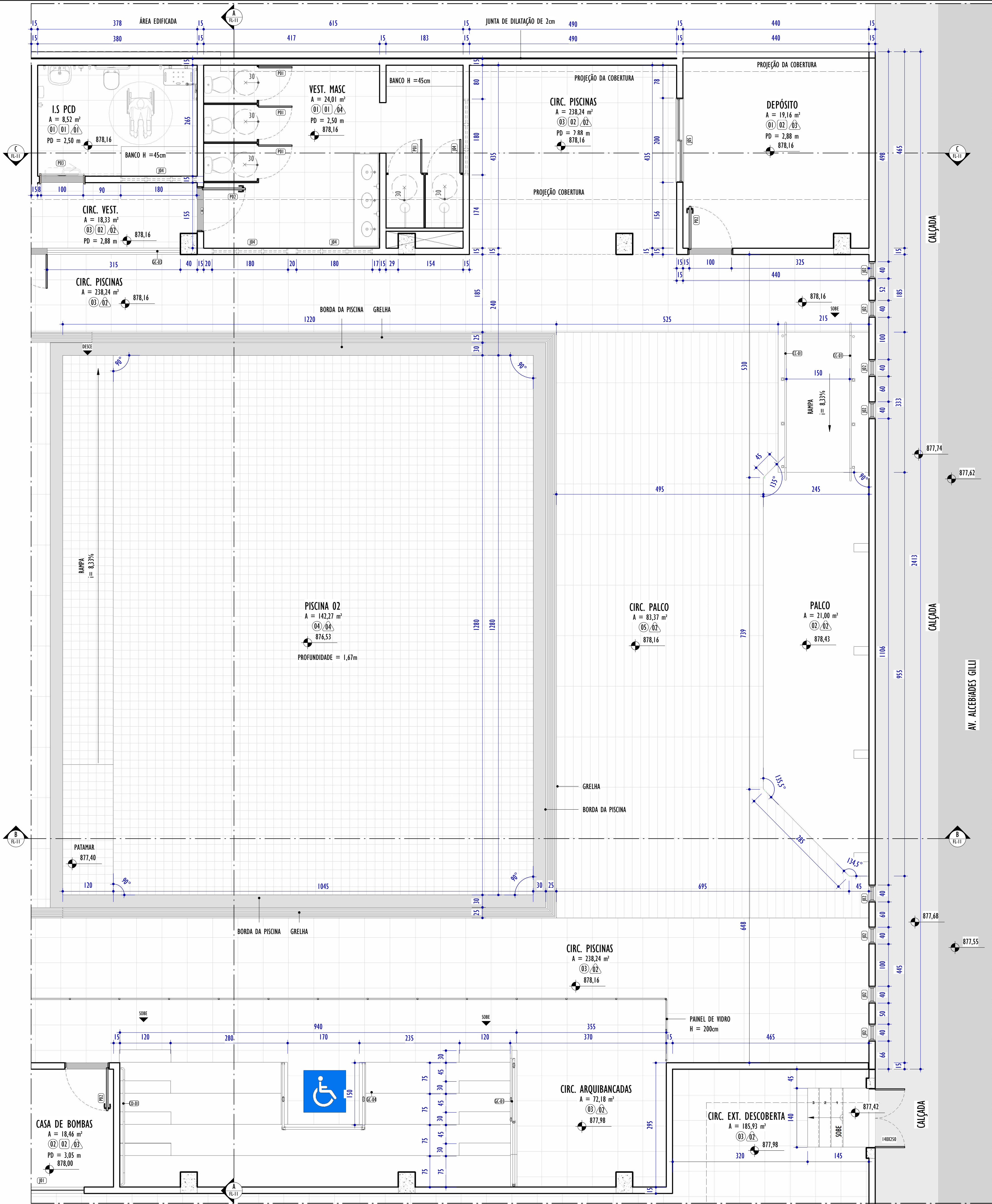
REFORMA - PLANTA - PARTE 02 ESCALA: 1 : 50
