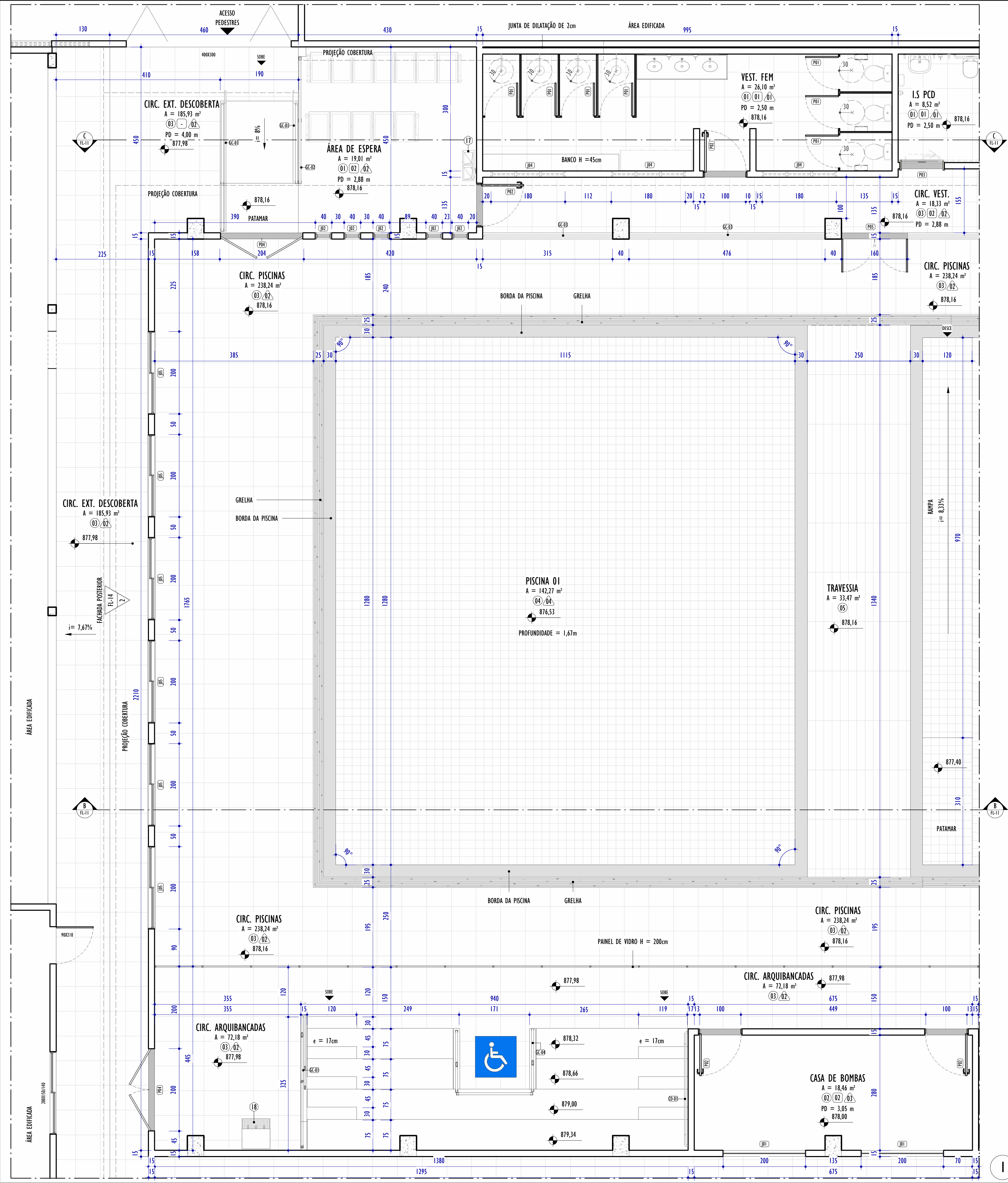
REFORMA - PLANTA - PARTE 01
