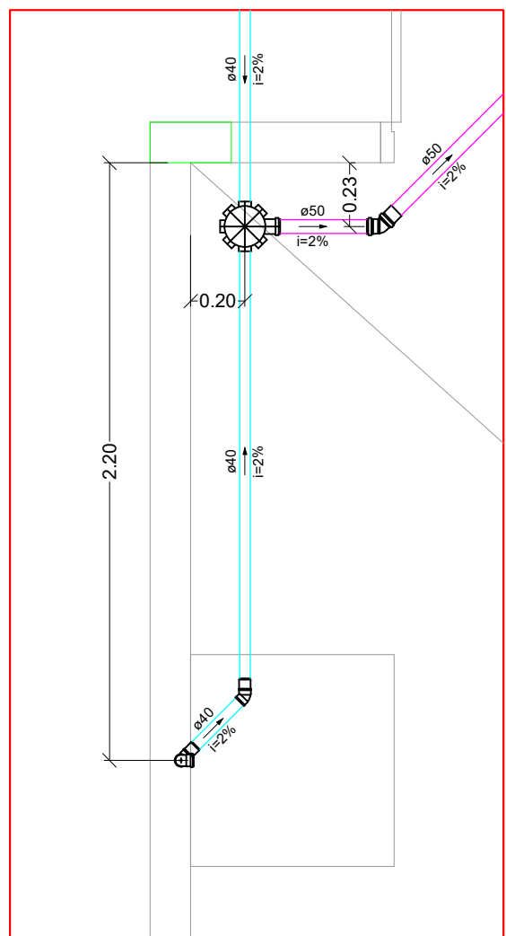
Detalhe S8 Escala 1:25
