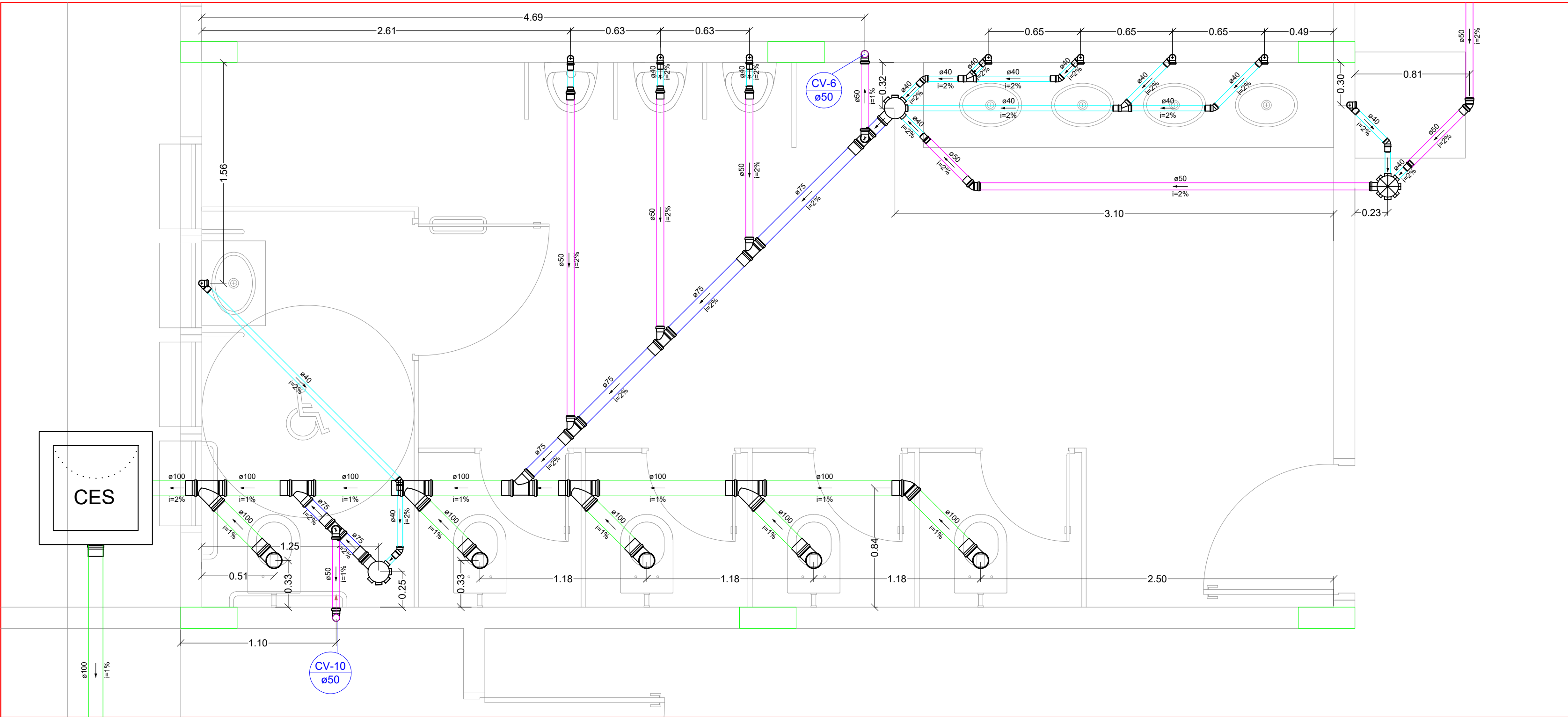
Detalhe S6 Escala 1:25
