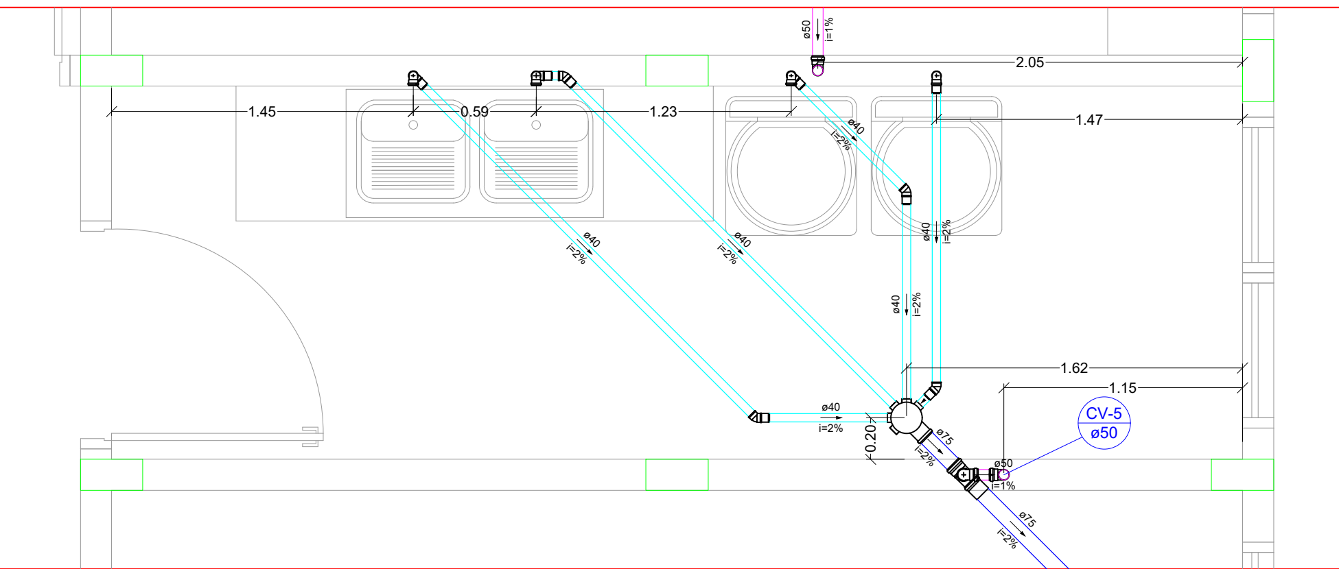
Detalhe S5 Escala 1:25
