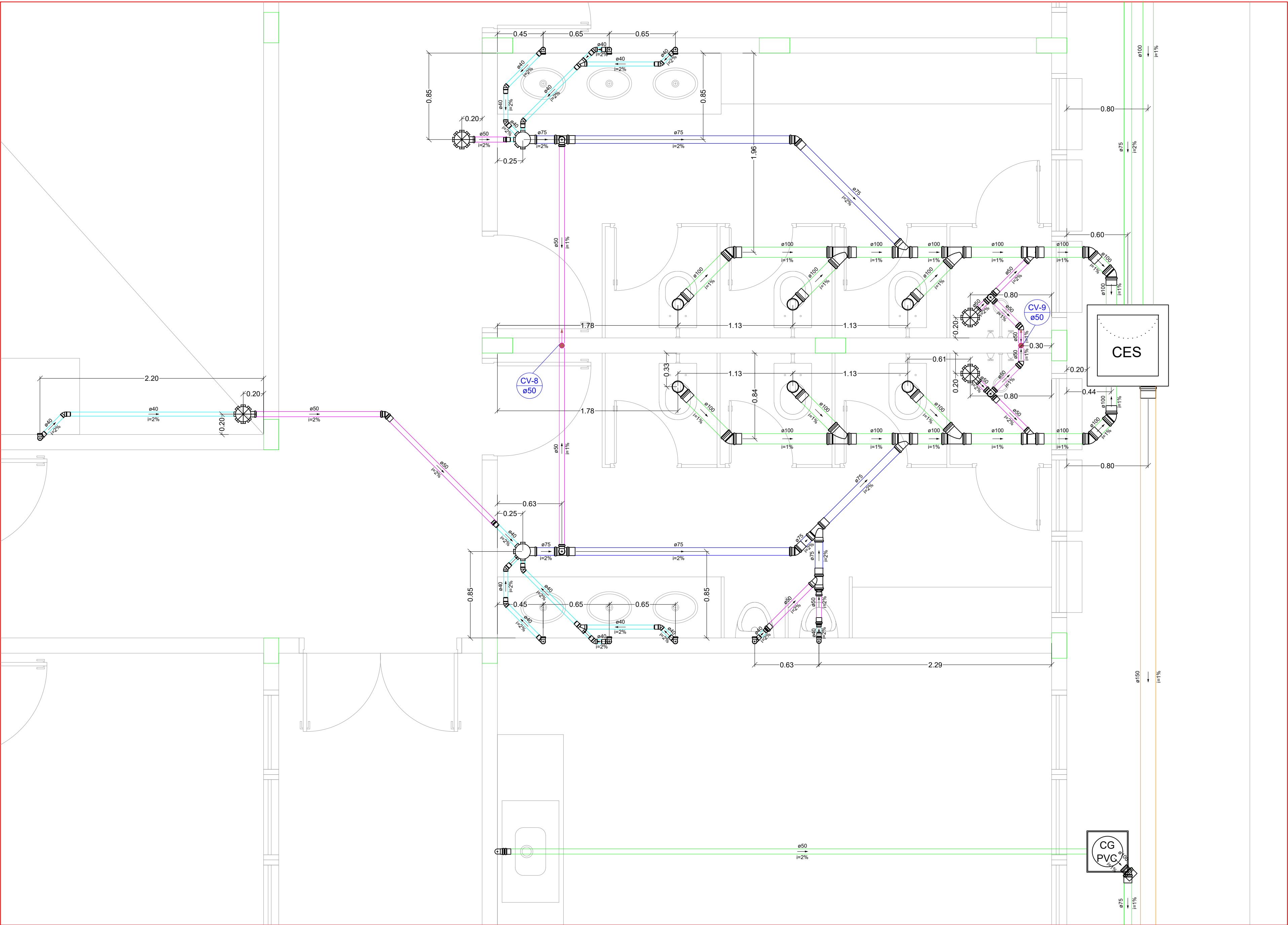
Detalhe S7 Escala 1:25
