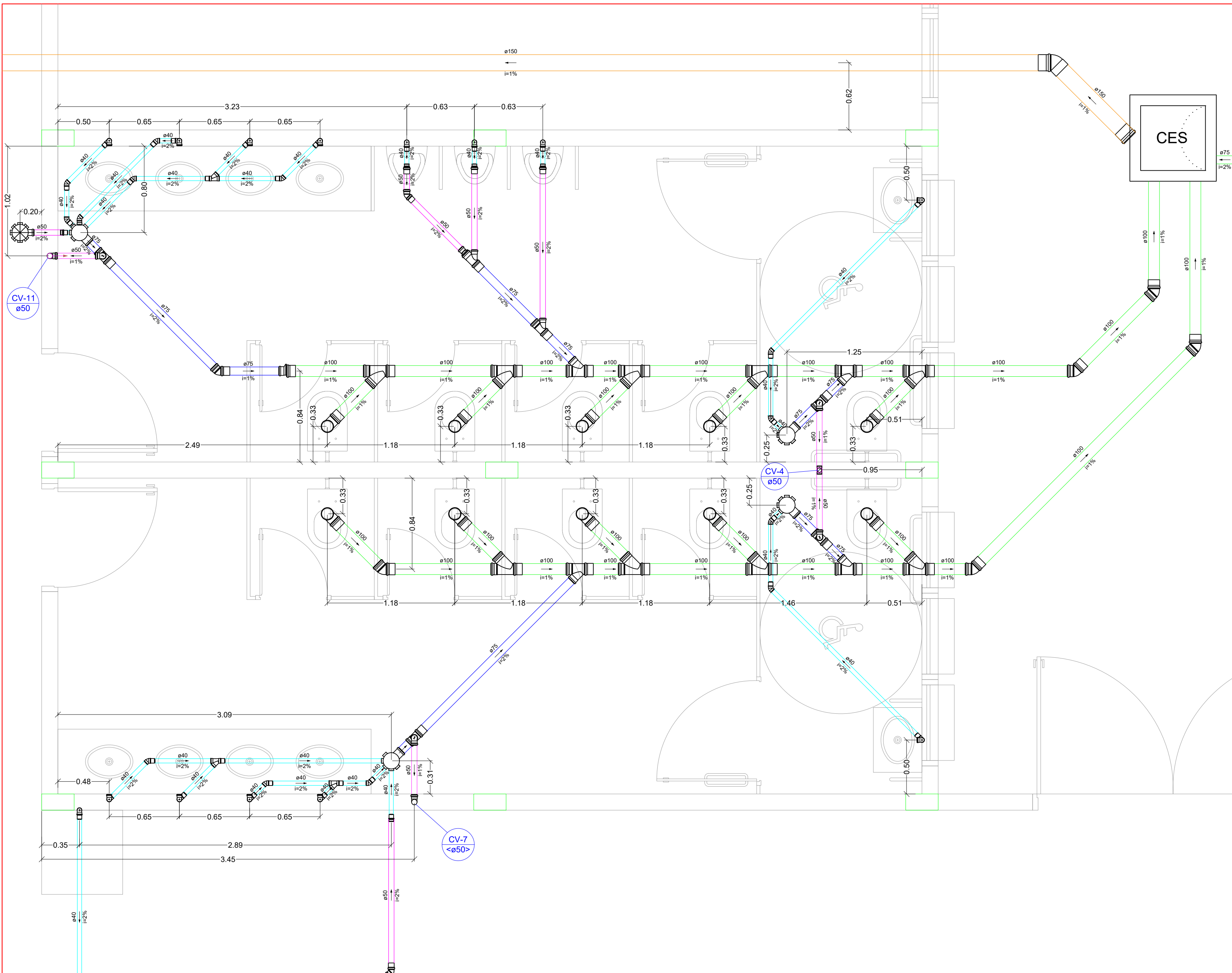
Detalhe S4 Escala 1:25
