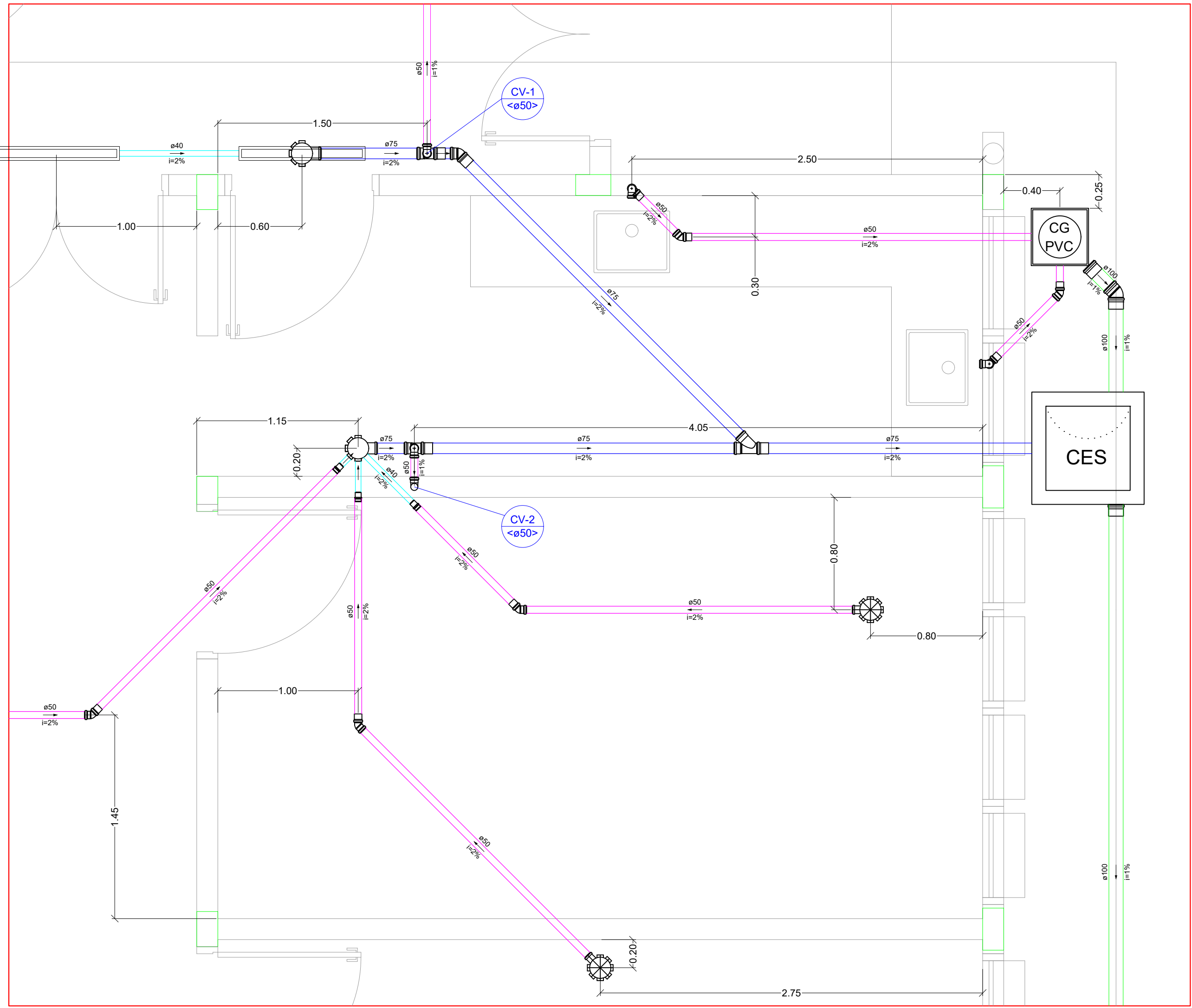
Detalhe S1 Escala 1:25
