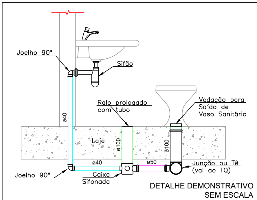
DETALHE DEMONSTRATIVO SEM ESCALA
