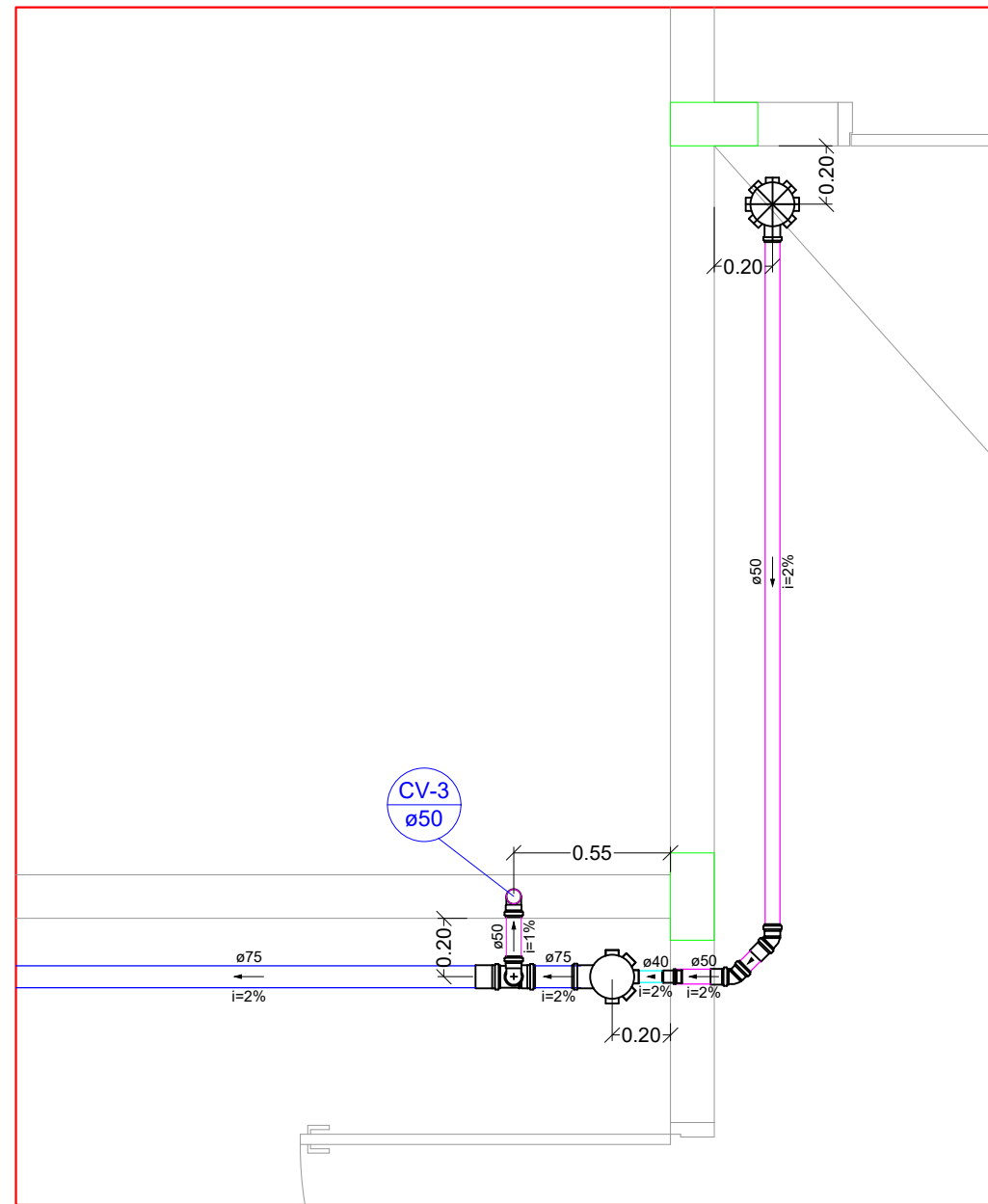
Detalhe S2 Escala 1:25
