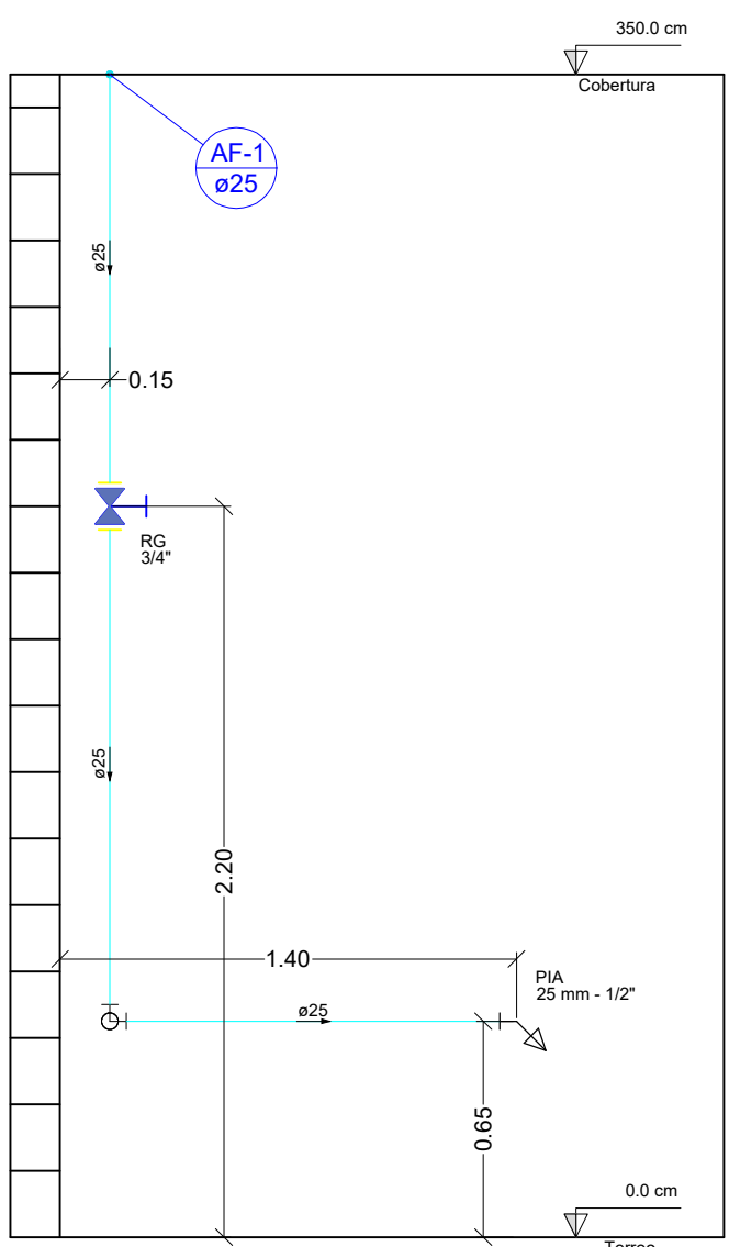
Detalhe H2 Escala 1:25
