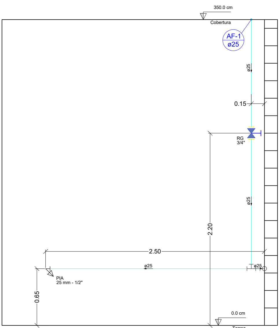
Detalhe H1 Escala 1:25
