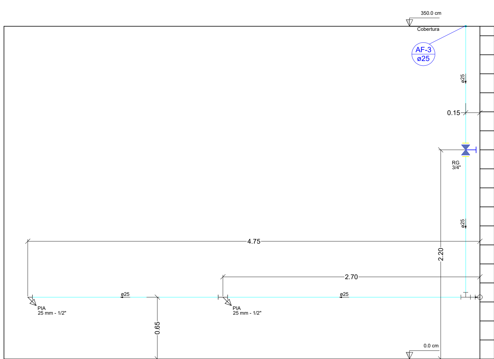
Detalhe H4 Escala 1:25
