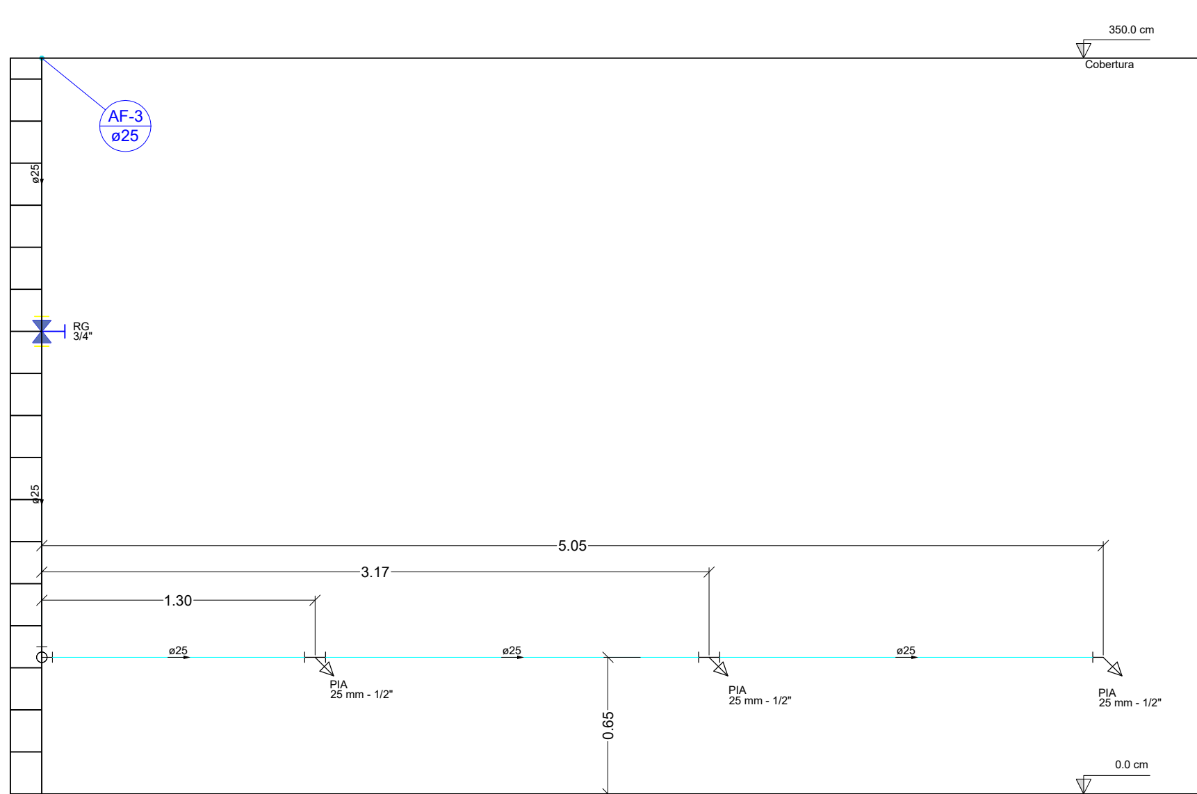
Detalhe H5 Escala 1:25
