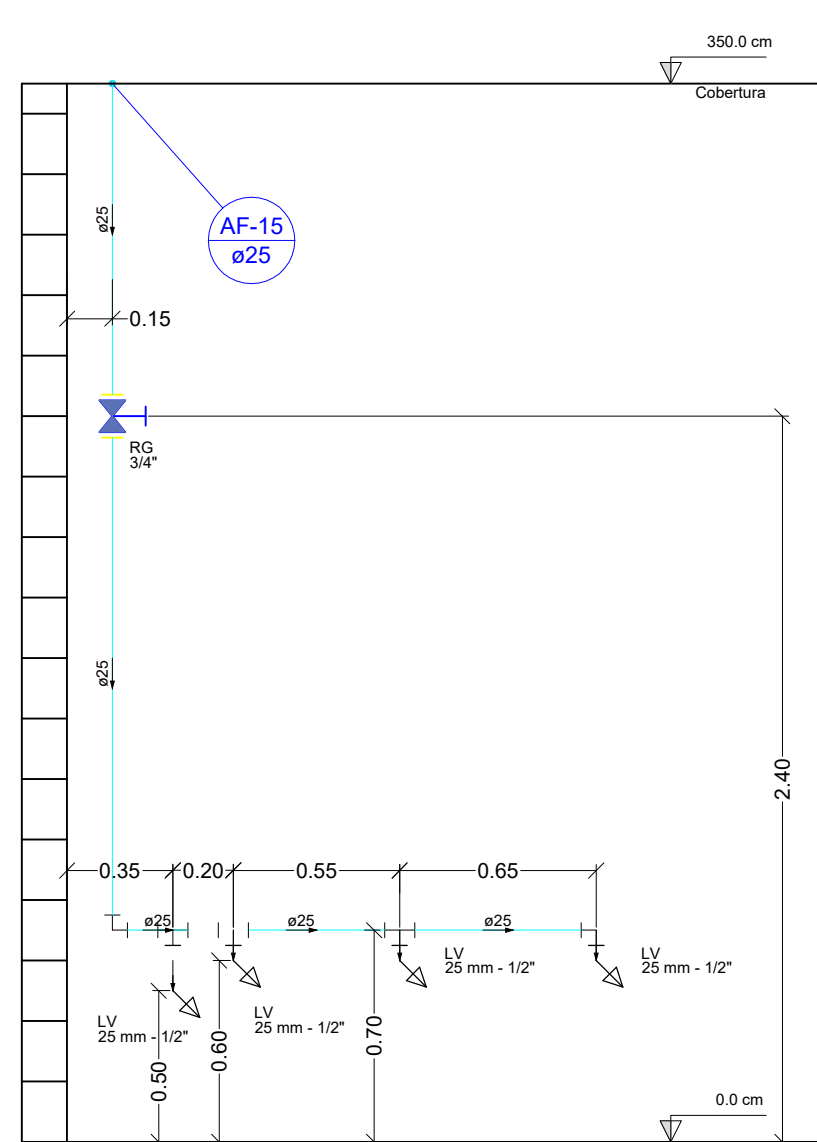
Detalhe H7 Escala 1:25
