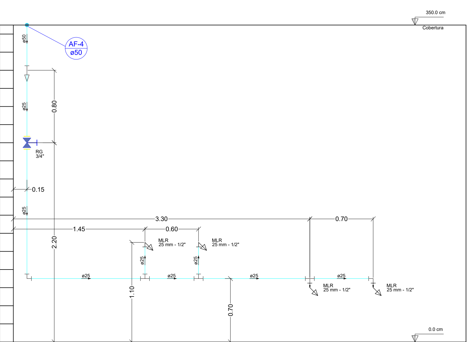
Detalhe H6 Escala 1:25
