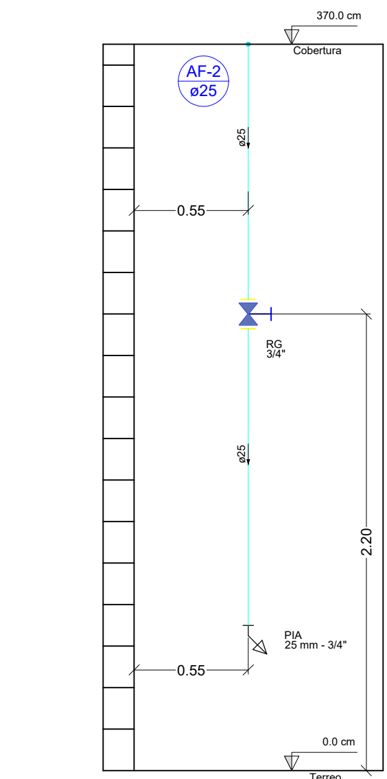
Detalhe H3 Escala 1:25
