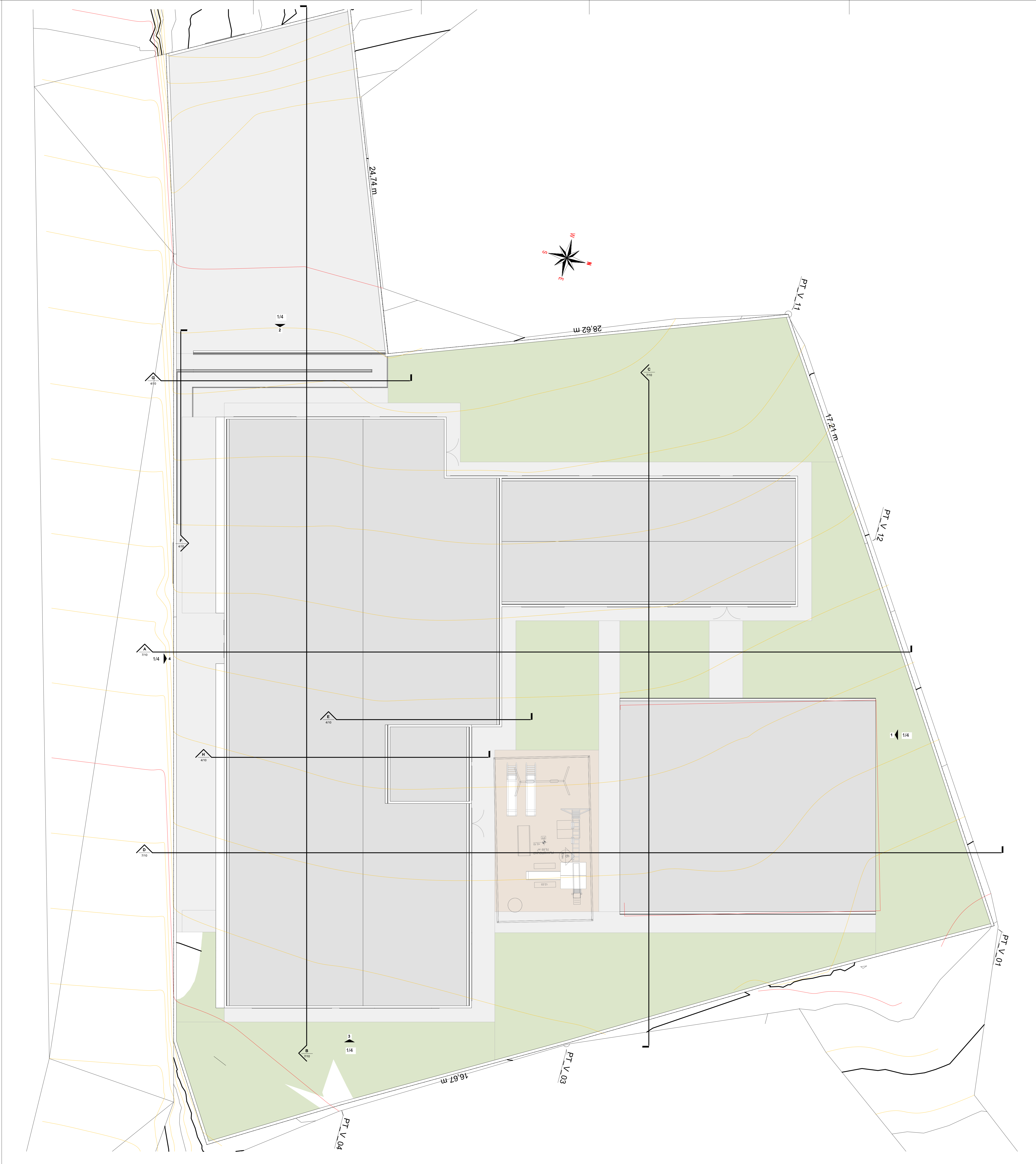
1 PLANTA REFERÊNCIA DE TOPOGRAFIA ESCALA: 1:100
