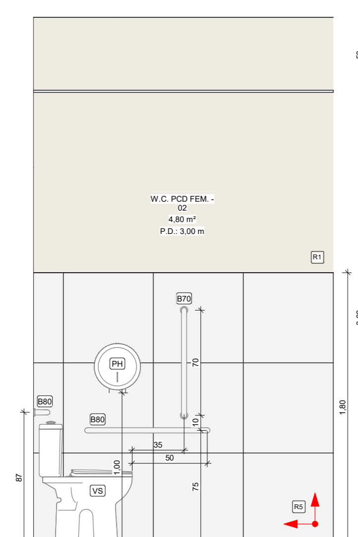
12 W.C. PCD FEM. 02 - VISTA B 1:25
