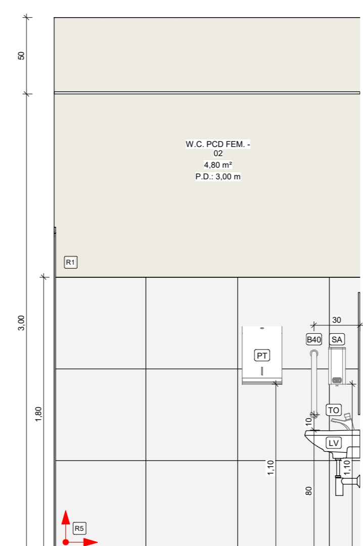
13 W.C. PCD FEM. 02 - VISTA C 1:25
