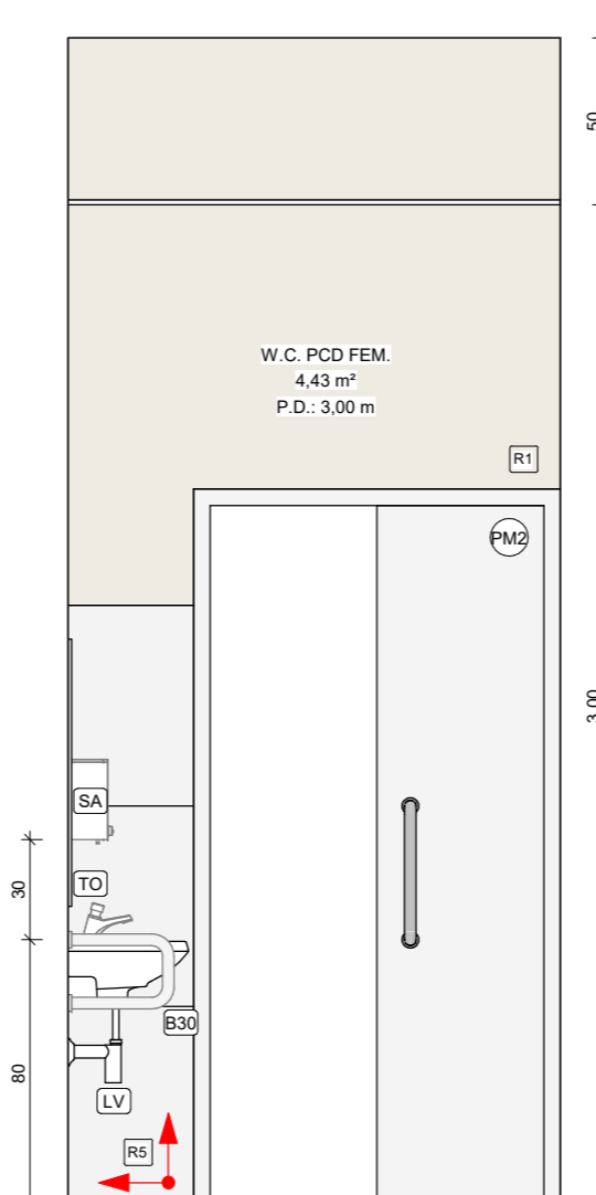
6 W.C. PCD FEM. 01 - VISTA B 1:25
