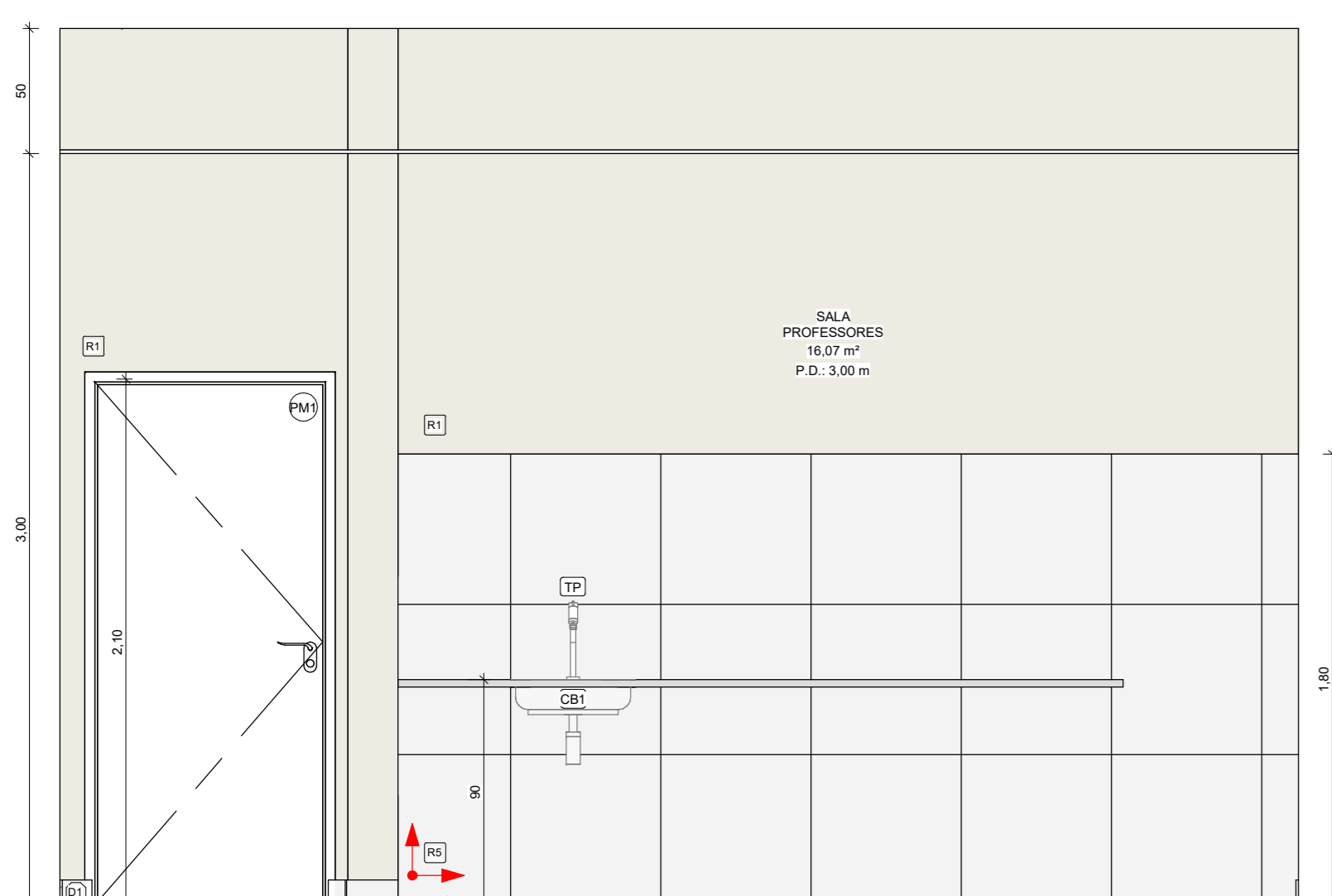
3 SALA PROFESSORES - VISTA A 1:25
