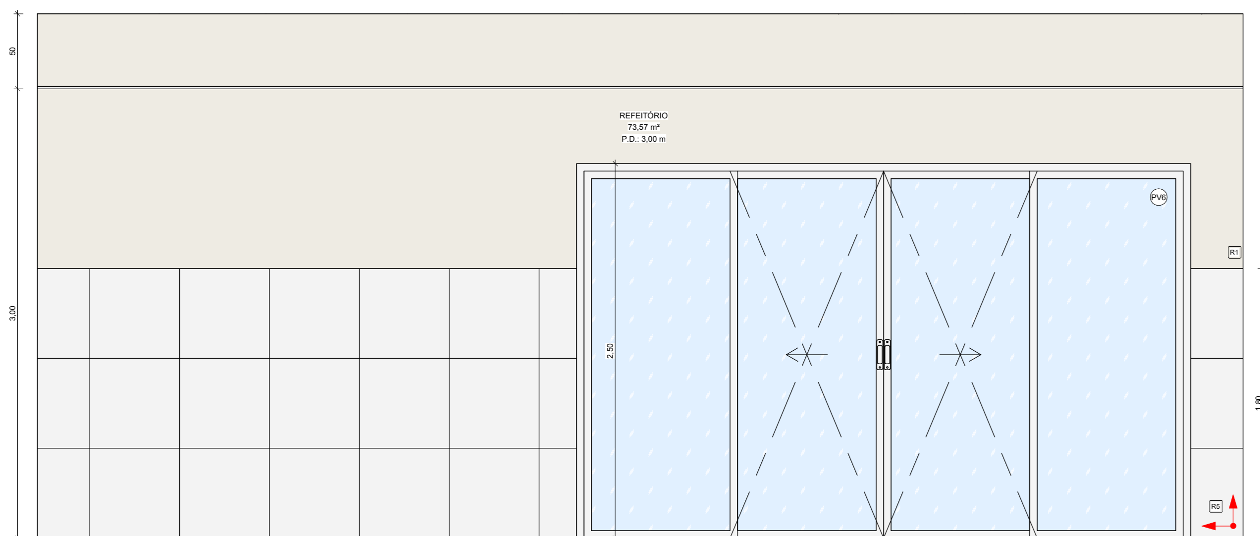
1 REFEITÓRIO - VISTA C 1:25
