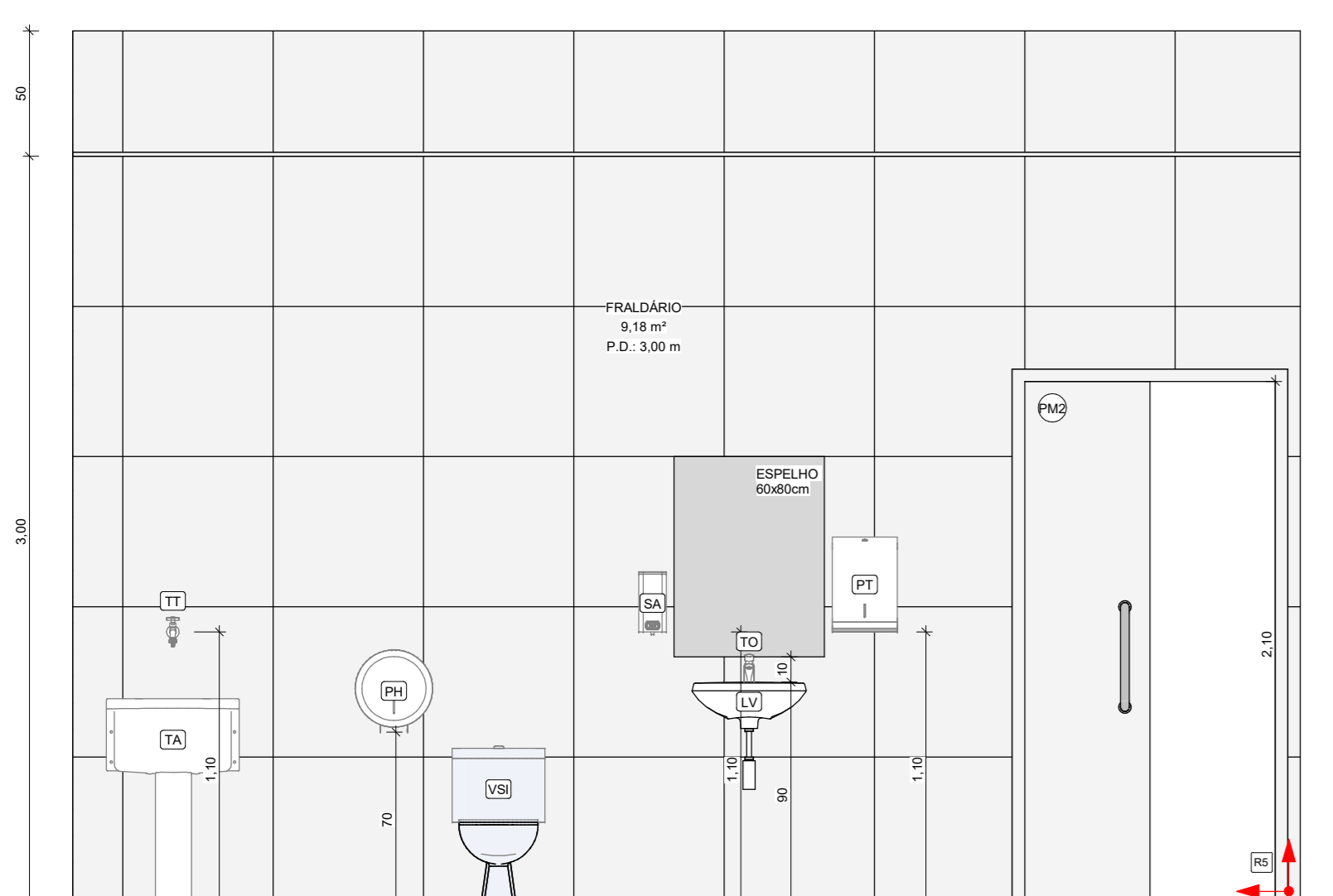
18 FRALDÁRIO - VISTA B 1:25
