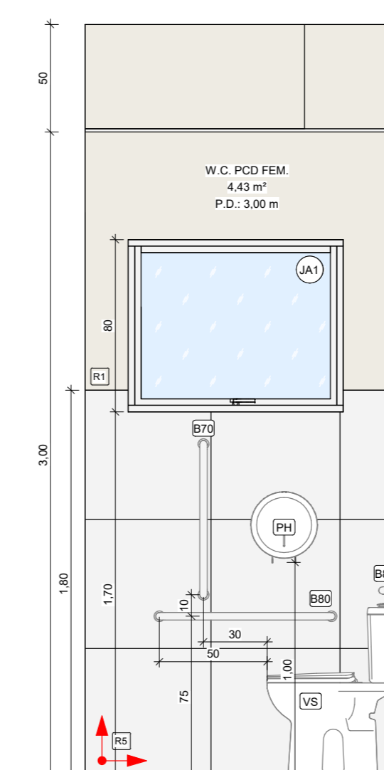
7 W.C. PCD FEM. 01 - VISTA C 1:25
