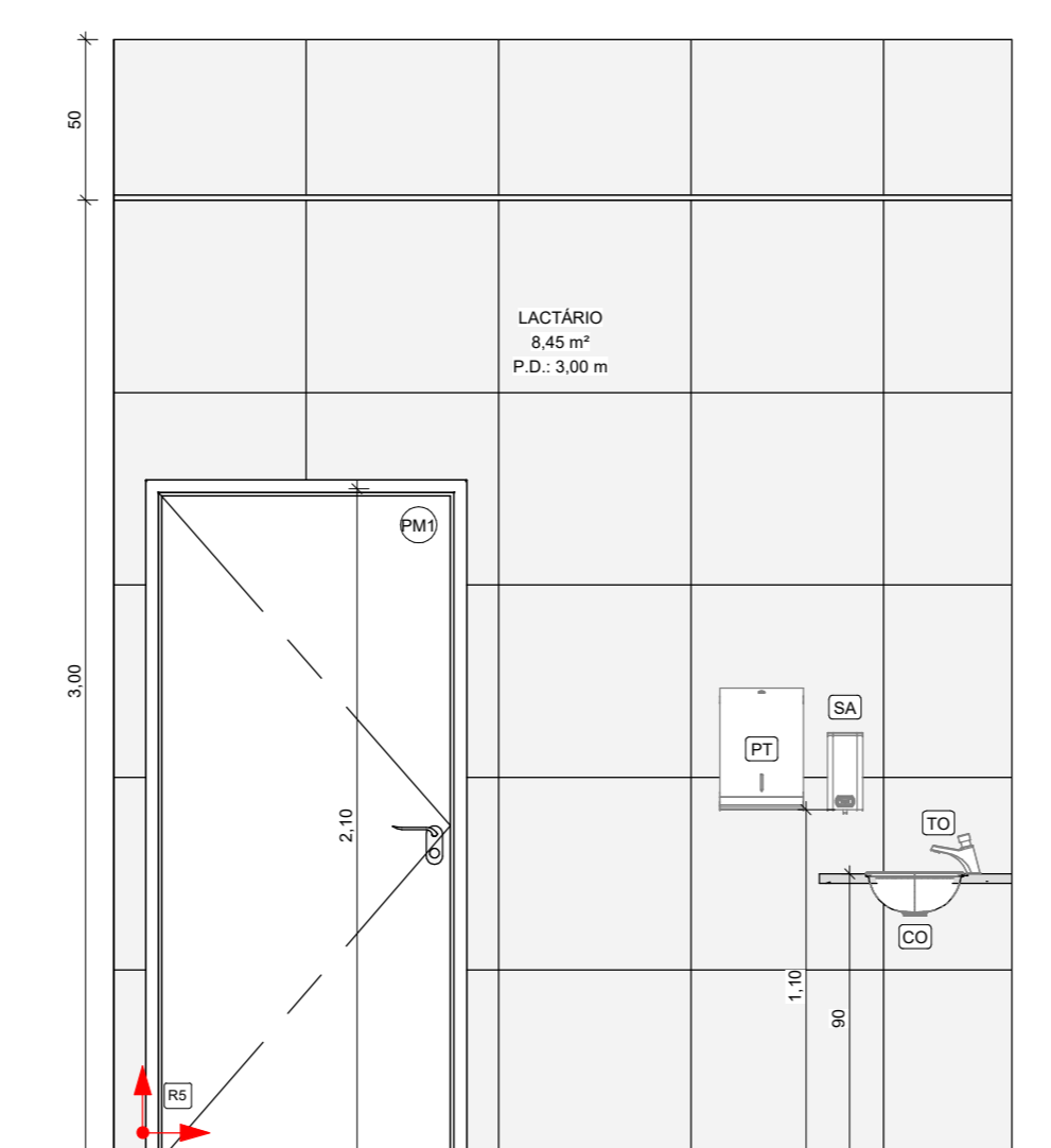
20 LACTÁRIO - VISTA A 1:25
