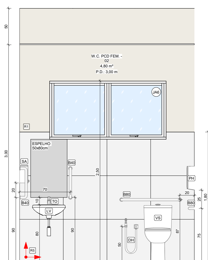
11 W.C. PCD FEM. 02 - VISTA A 1:25
