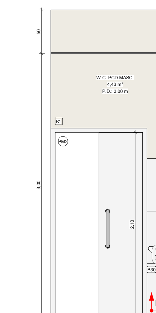
9 W.C. PCD MASC. 01 - VISTA B 1:25
