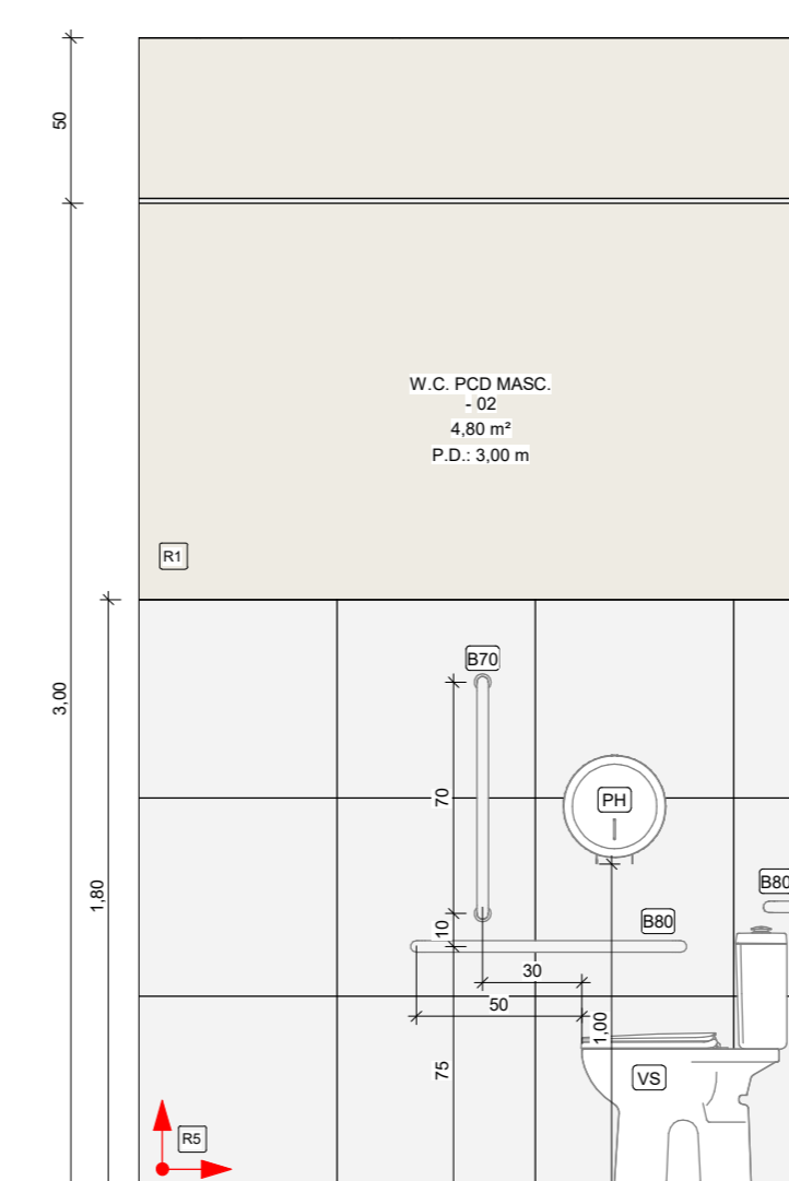
16 W.C. PCD MASC. 02 - VISTA C 1:25
