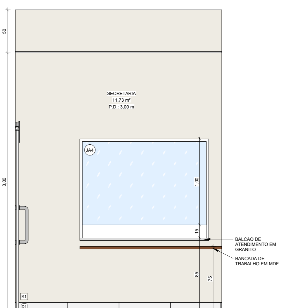
4 SECRETARIA - VISTA A 1:25
