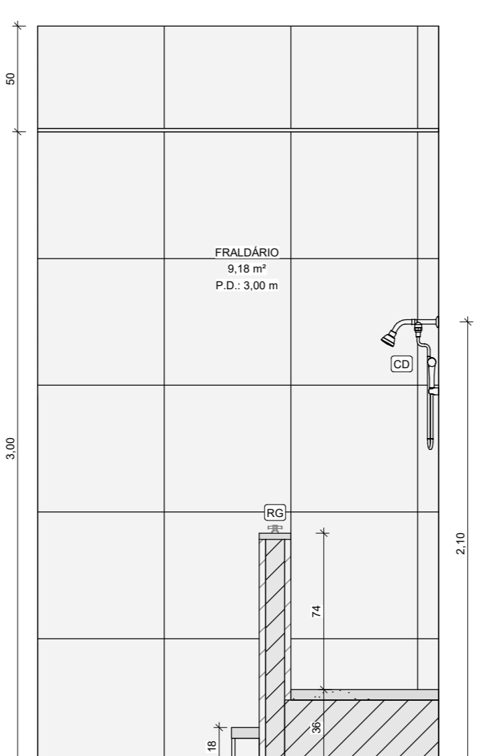
19 FRALDÁRIO - VISTA C 1:25
