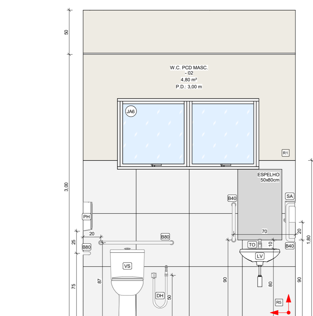
14 W.C. PCD MASC. 02 - VISTA A 1:25
