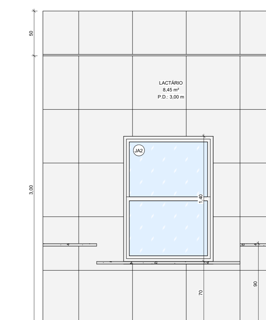
22 LACTÁRIO - VISTA C 1:25
