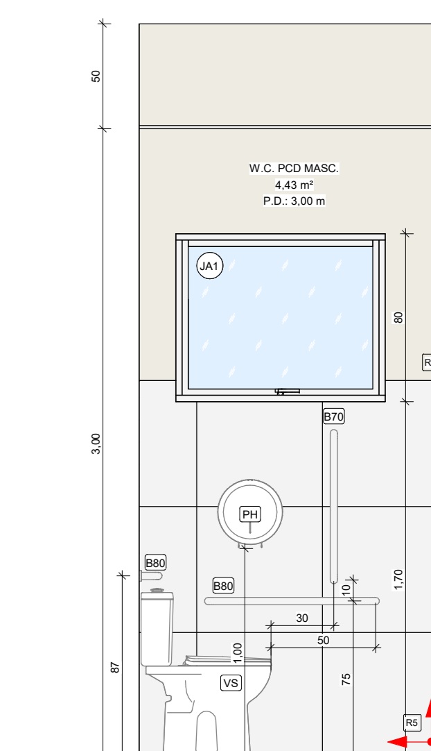
10 W.C. PCD MASC. 01 - VISTA C 1:25
