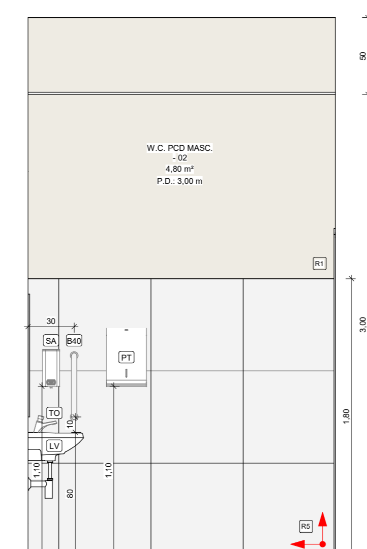
15 W.C. PCD MASC. 02 - VISTA B 1:25
