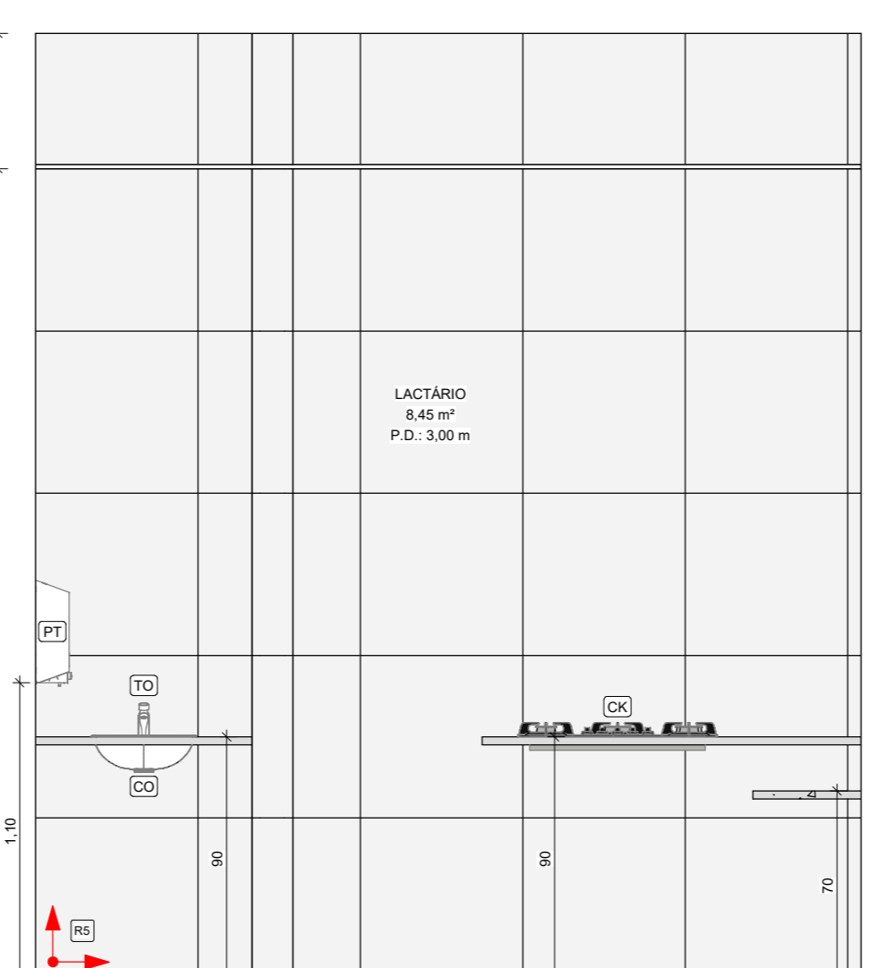
21 LACTÁRIO - VISTA B 1:25
