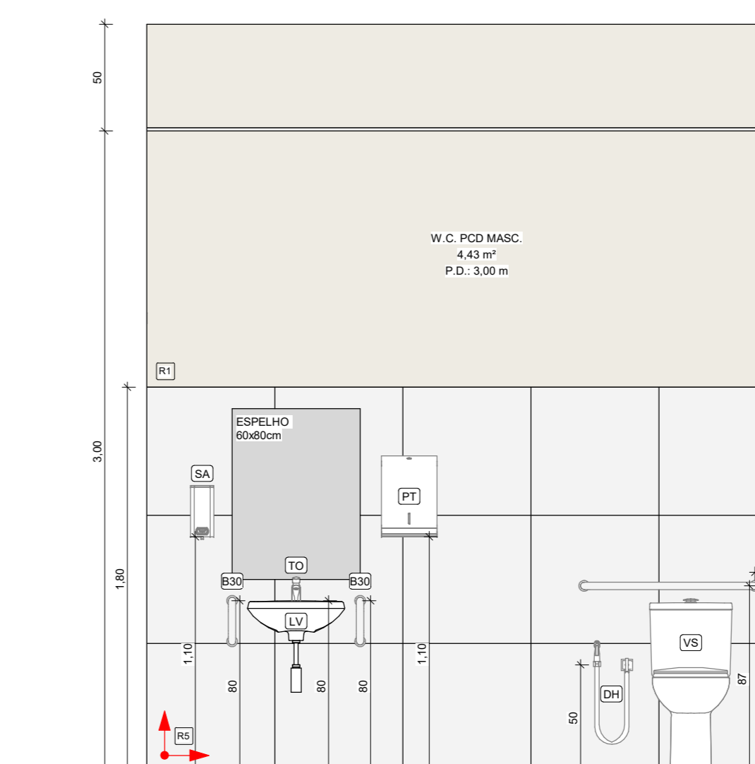
8 W.C. PCD MASC. 01 - VISTA A 1:25
