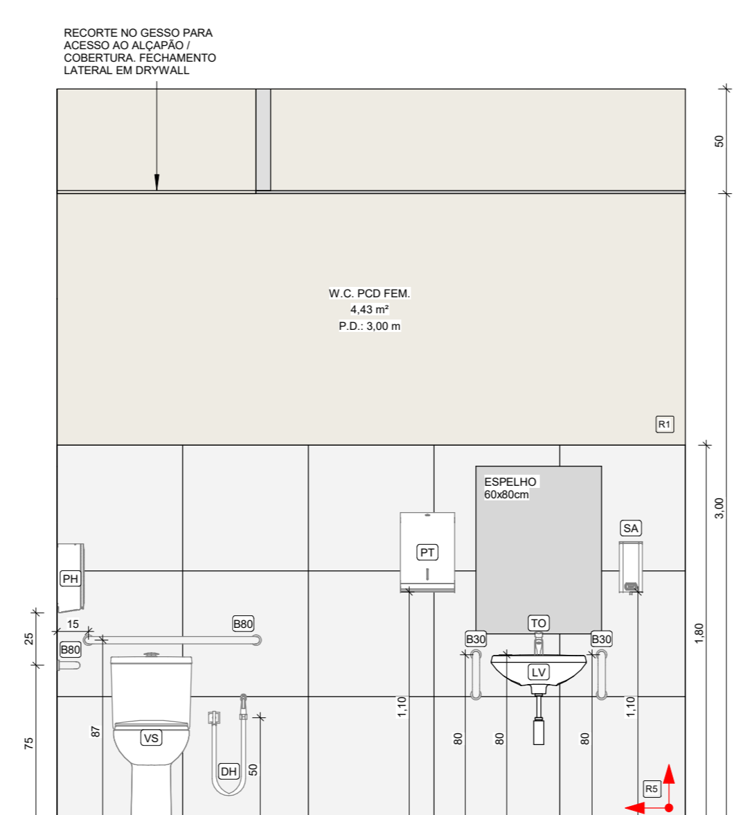
5 W.C. PCD FEM. 01 - VISTA A 1:25
