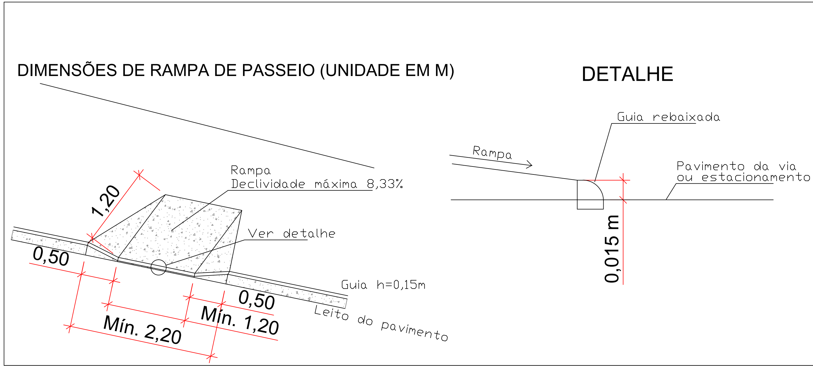
DETALHE - RAMPA DE ACESSIBILIDADE S/ ESCALA
