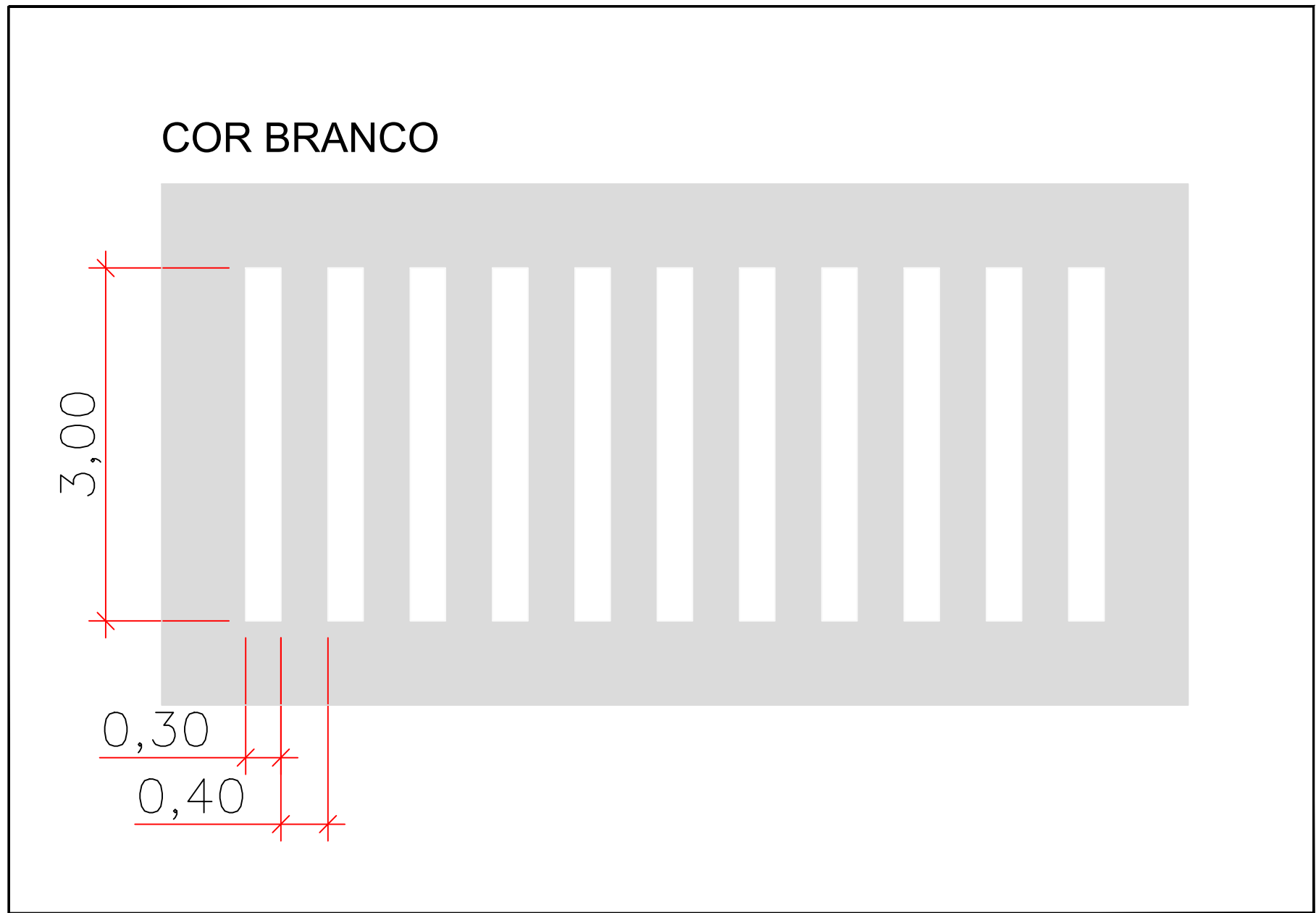
DETALHE - FAIXA DE PEDESTRE S/ ESCALA
