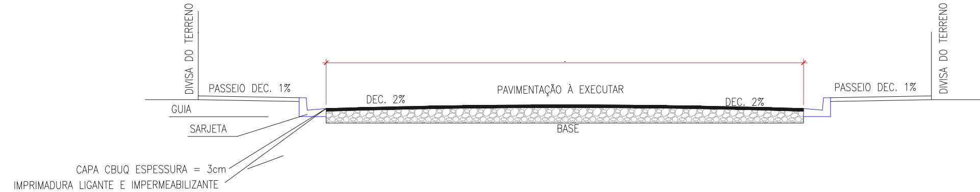
SEÇÃO TÍPICA DO RECAPEAMENTO COM ESPESSURA DE CBUQ DE 3 CM SEM ESCALA
