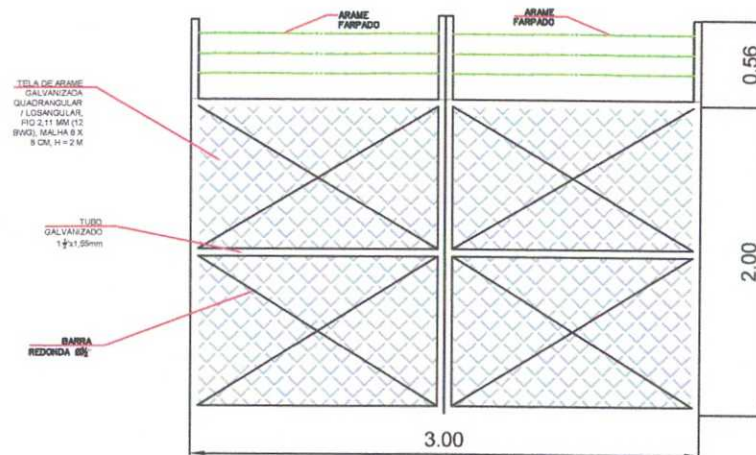
PORTÃO S/ESC.
