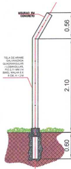
CORTE S/ESC.
