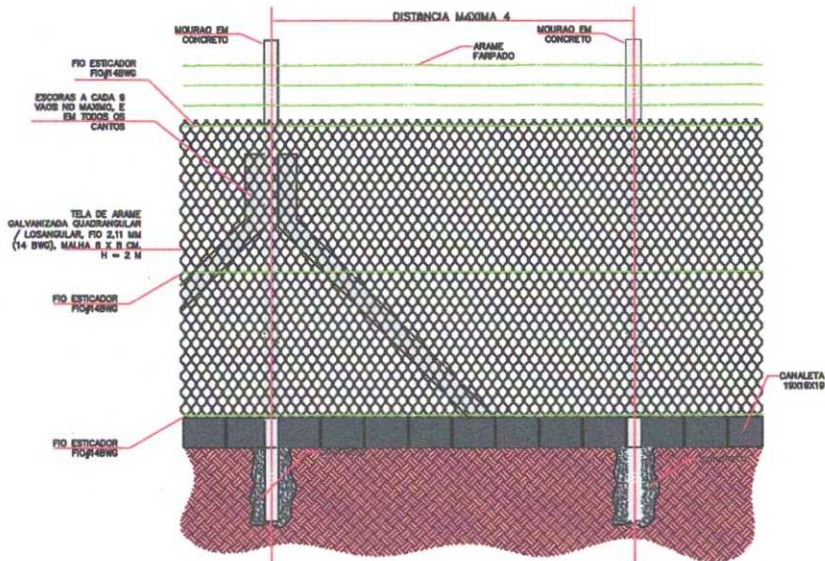
ELEVAÇÃO DO ALAMBRADO S/ESC.
