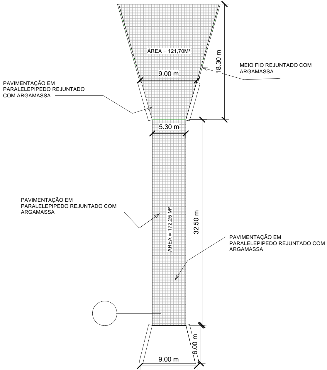
1 Planta baixa 1 : 300
