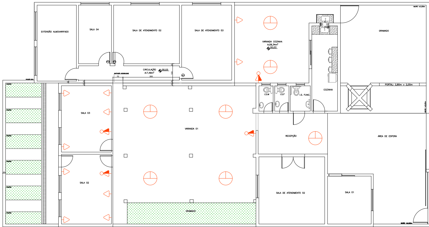
PLANTA PONTOS ELÉTRICOS ESC:1-150
