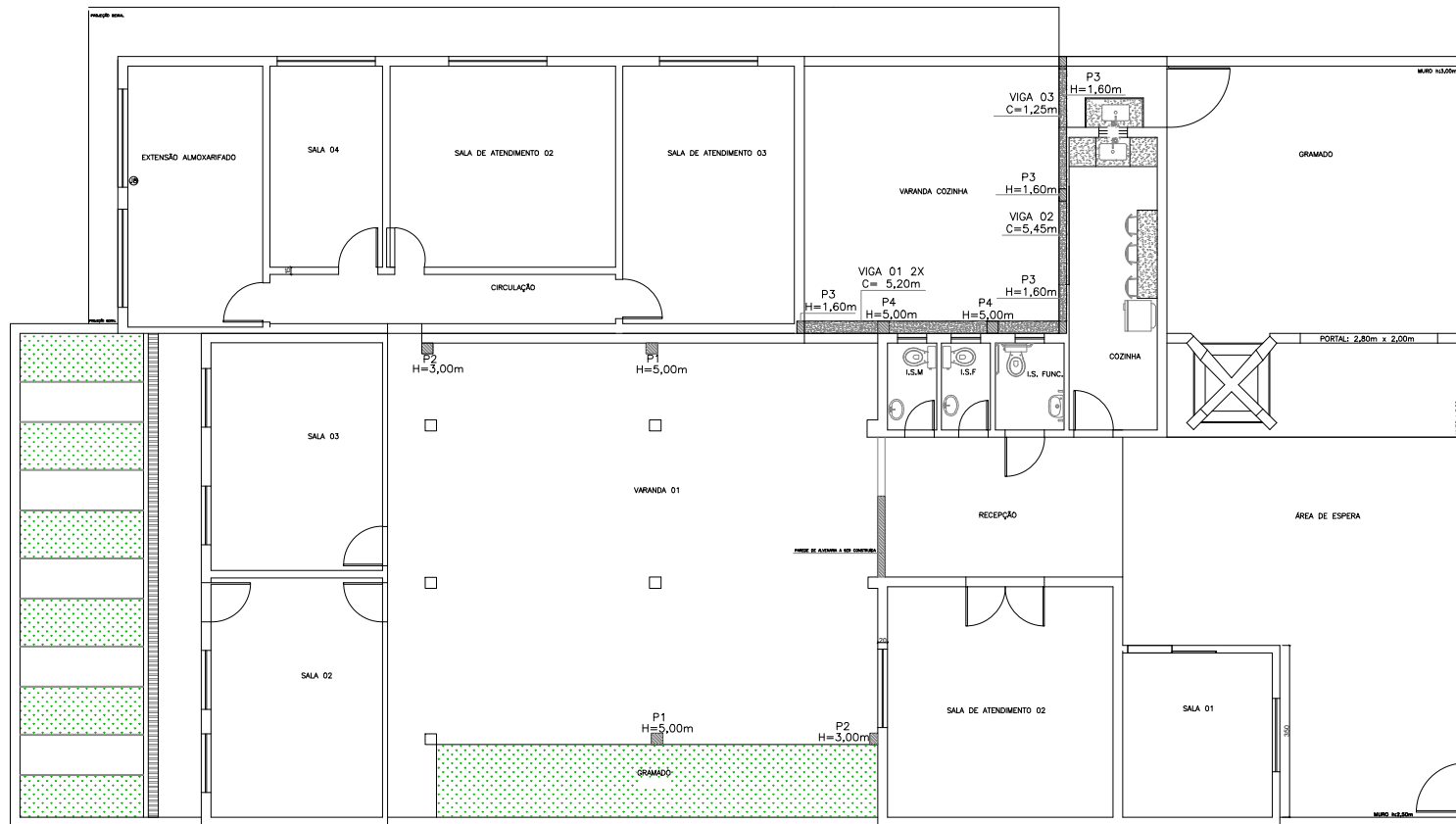
LOCAÇÃO PILARES E VIGAS ESC:1-150
