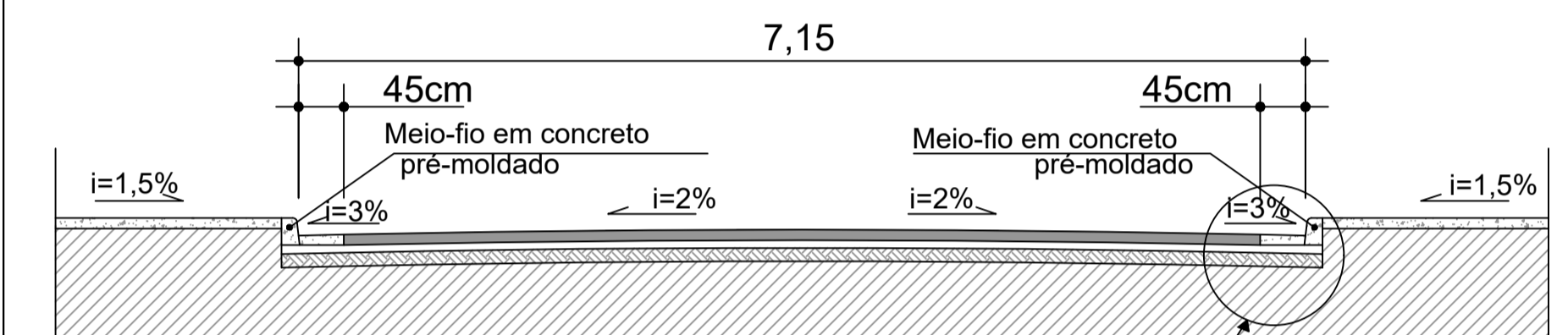
SEÇÃO TÍPICA RUA IBITURUNA (PAV. EXIST.: POLIEDRO)
