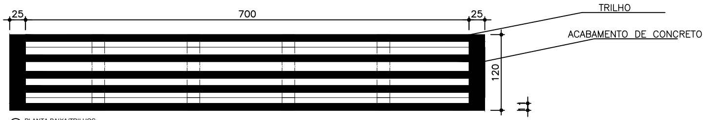
1 PLANTA BAIXA/TRILHOS
