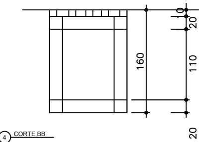
4 CORTE BB
