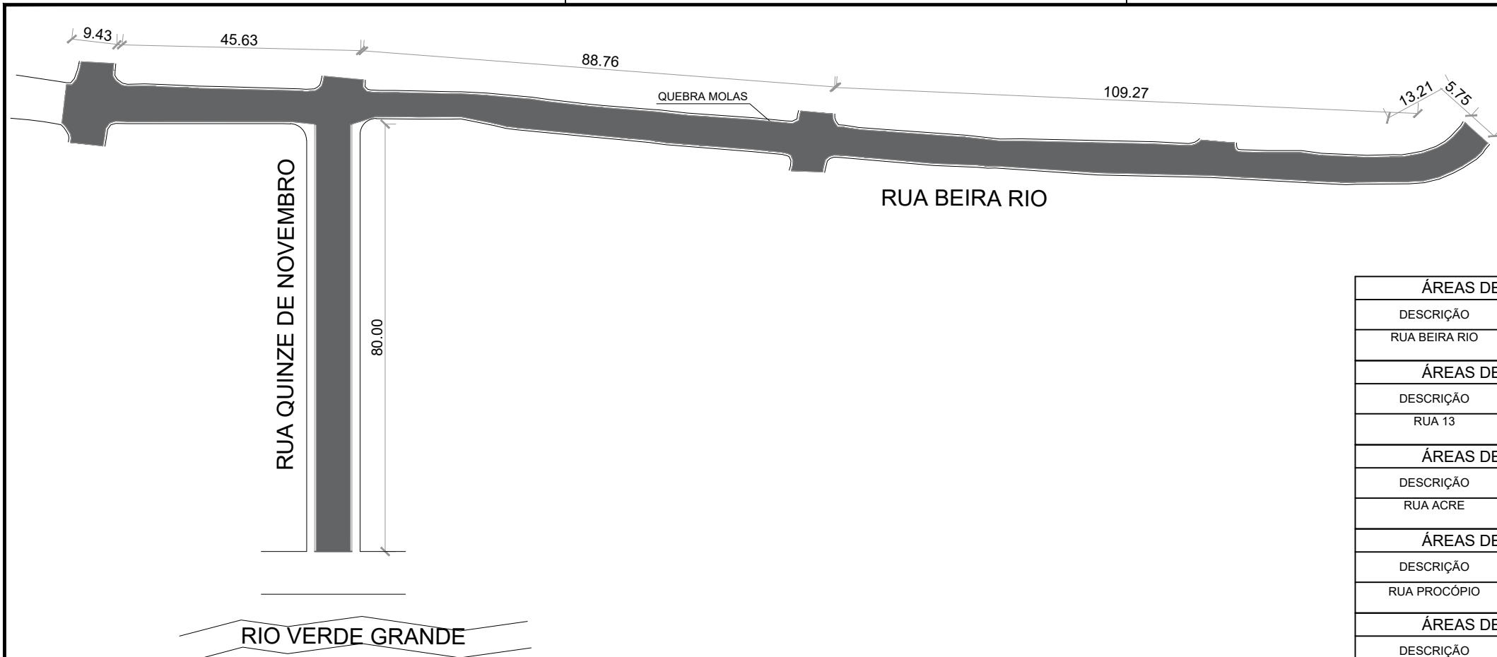
Projeto de pavimentação esc. 1:1000
