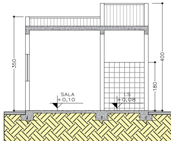
Corte BB sem escala
