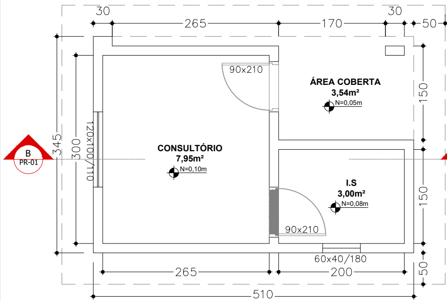
Planta Baixa Cotada sem escala
