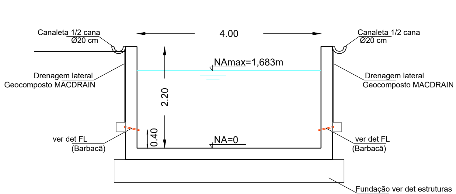
DETALHE DOS ELEMENTOS
