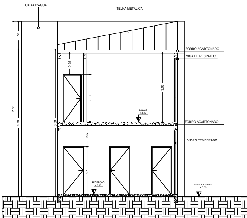
6 CORTE AA ESCALA.....1/50
