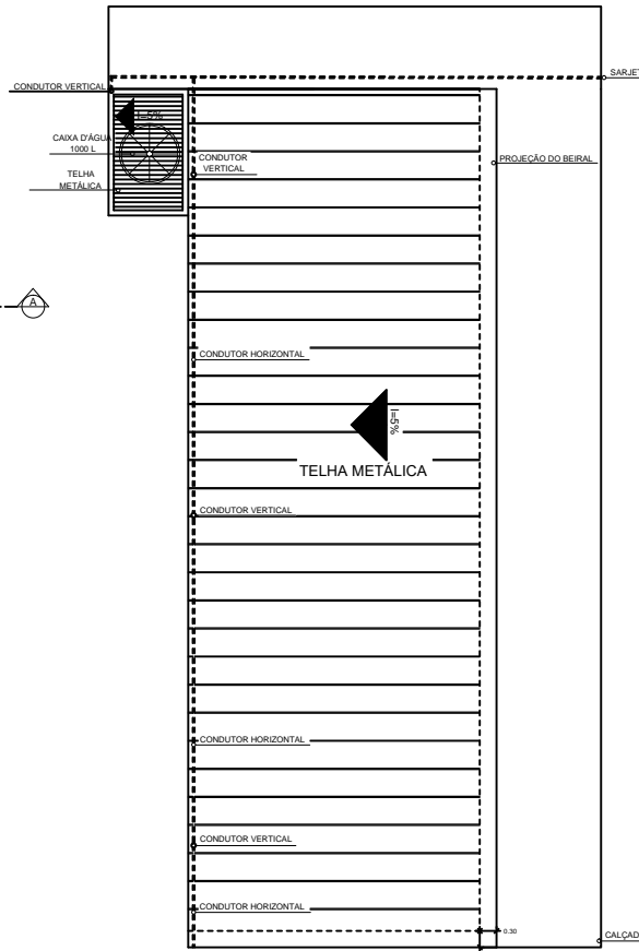
3 PLANTA DE COBERTURA ESCALA.....1/75
