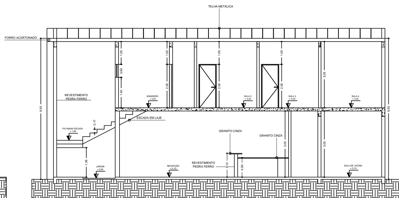
7 CORTE BB ESCALA.....1/50
