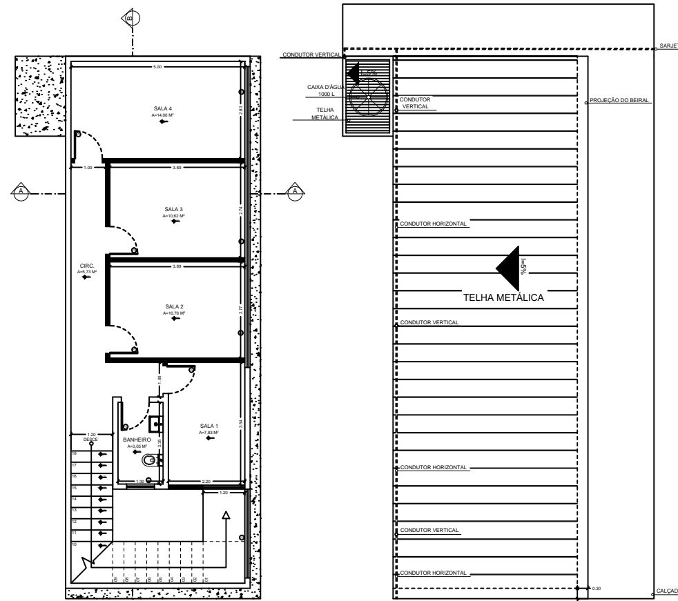
2 PLANTA BAIXA 1º PAVIMENTO ESCALA.....1/75
