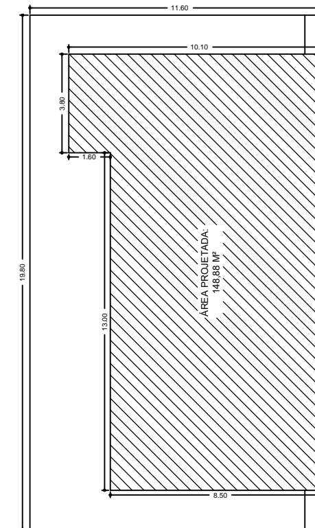
4 IMPLANTAÇÃO ESCALA.....1/100
