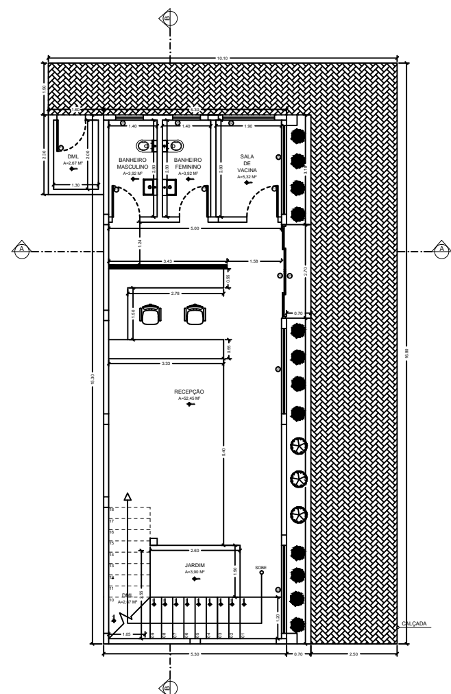
1 PLANTA BAIXA TÉRREO ESCALA.....1/75
