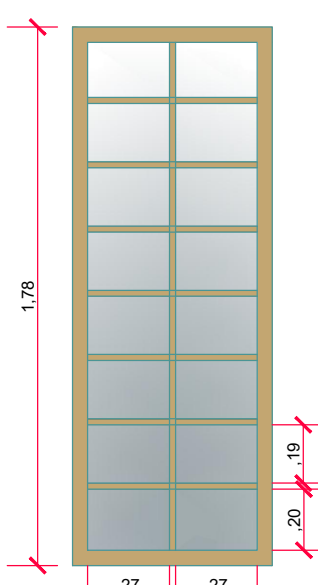
VISTA FRONTAL: JANELA 10 - fixa/ basculante - FERRO/ VIDRO Escala 1: 25
