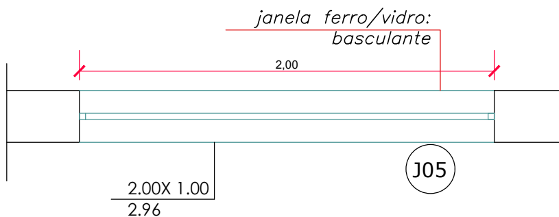
PLANTA-BAIXA: JANELA 05 - fixa/ basculante FERRO/ VIDRO Escala 1: 25
