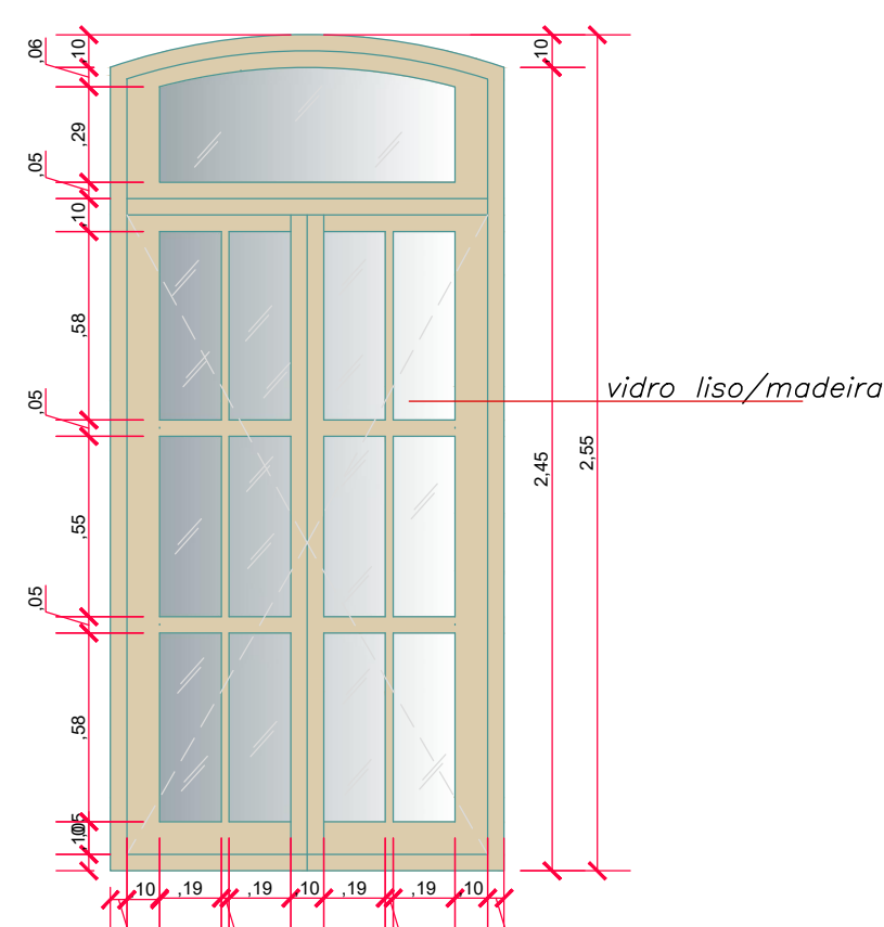
VISTA FRONTAL: JANELA 02 - ABRIR VIDRO / MADEIRA Escala 1: 25
