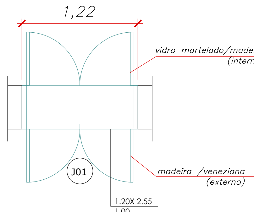
PLANTA-BAIXA: JANELA 01 - ABRIR VENEZIANA (MADEIRA)/ VIDRO MARTELADO Escala 1: 25
