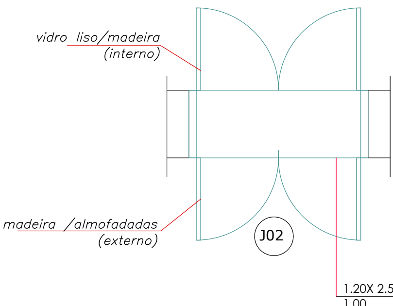
PLANTA-BAIXA: JANELA 02 - ABRIR PAINEL (MADEIRA)/ VIDRO LISO Escala 1: 25
