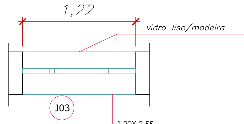
PLANTA-BAIXA: JANELA 03 - VIDRO LISO / MADEIRA Escala 1:25
