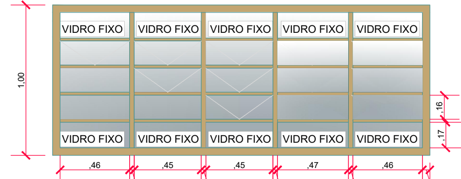
VISTA FRONTAL: JANELA 06 - fixa/ basculante FERRO/ VIDRO Escala 1: 25
