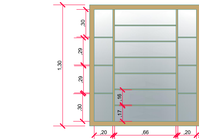
VISTA FRONTAL: JANELA 08 - fixa/ basculante - FERRO/ VIDRO Escala 1: 25
