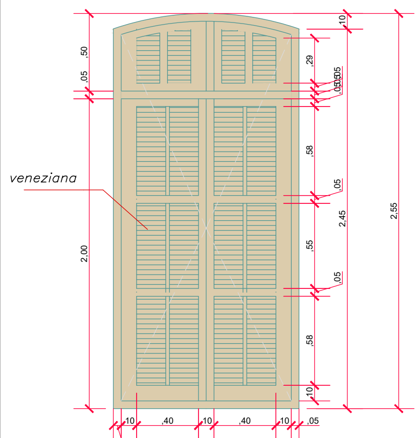
VISTA FRONTAL: JANELA 01 - ABRIR VENEZIANA (MADEIRA) Escala 1: 25
