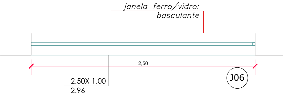
PLANTA-BAIXA: JANELA 06 - fixa/ basculante FERRO/ VIDRO Escala 1: 25
