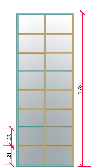
VISTA FRONTAL: JANELA 12 - fixa/ basculante - FERRO/ VIDRO
