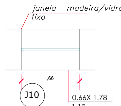
PLANTA-BAIXA: JANELA 10 - fixa/ basculante - FERRO/ VIDRO Escala 1: 25
