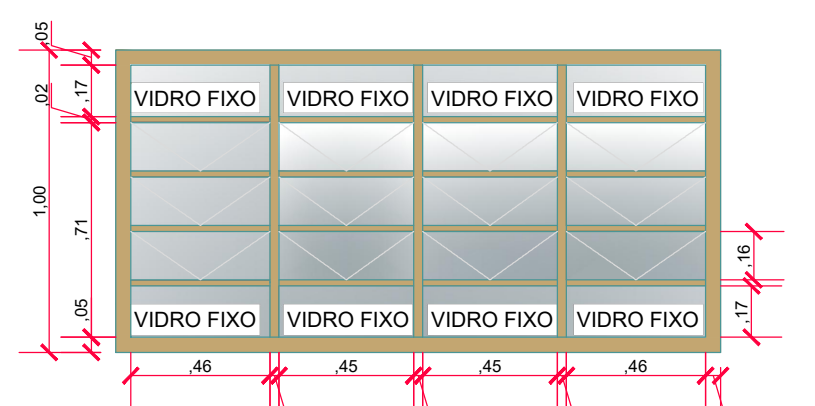
VISTA FRONTAL: JANELA 05 - fixa/ basculante FERRO/ VIDRO Escala 1: 25
