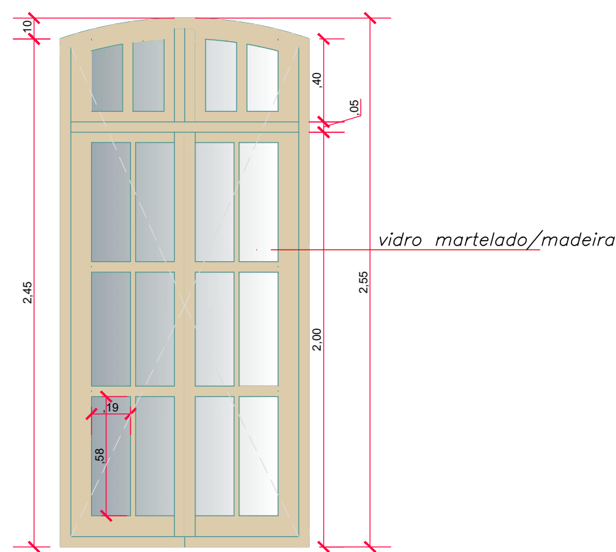
VISTA FRONTAL: JANELA 01 - ABRIR VIDRO /MADEIRA Escala 1: 25
