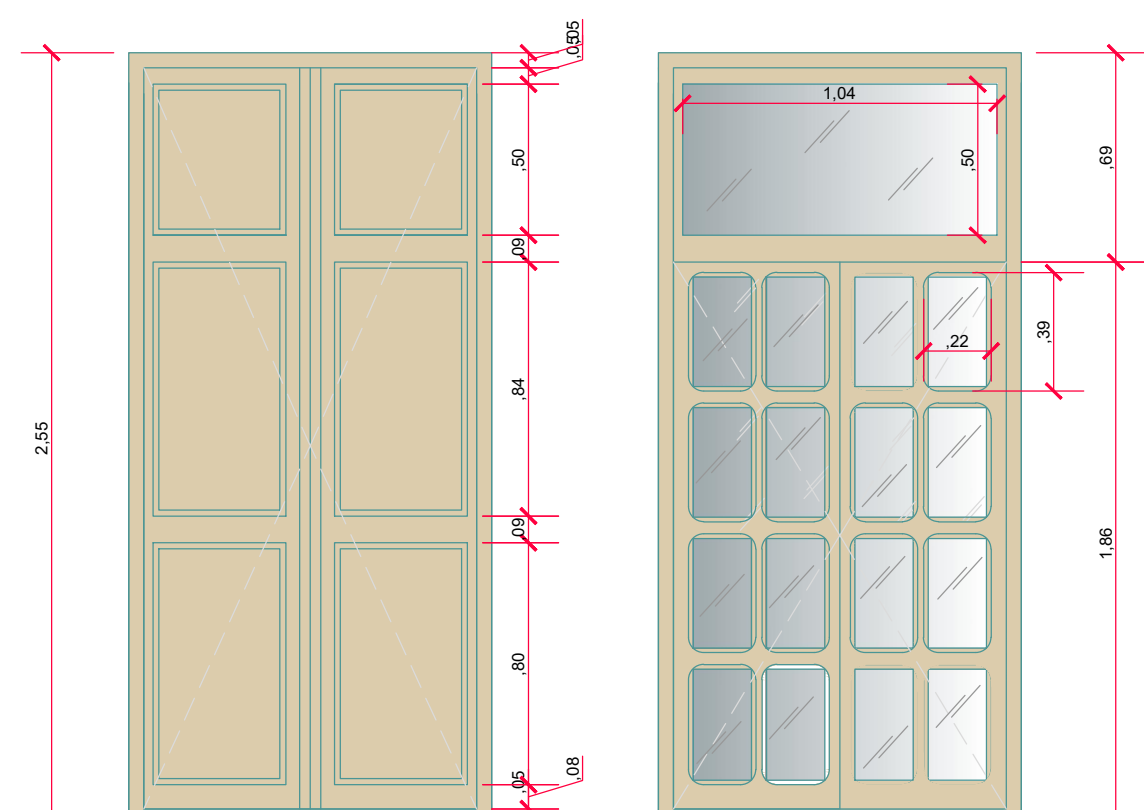
VISTA FRONTAL: JANELA 04 - ABRIR PAINEL (MADEIRA)/ VIDRO MARTELADO Escala 1: 25
