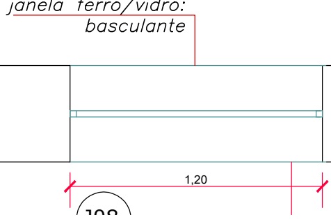
PLANTA-BAIXA: JANELA 08 - fixa/ basculante - FERRO/ VIDRO Escala 1: 25
