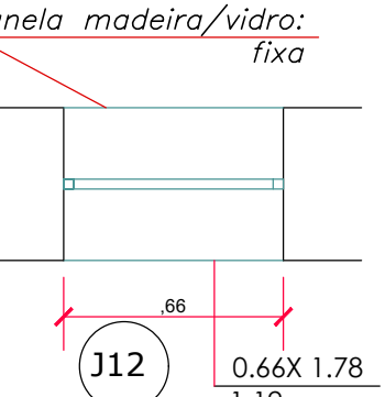
PLANTA-BAIXA: JANELA 12 - fixa/ basculante - MADEIRA/ VIDRO Escala 1: 25
