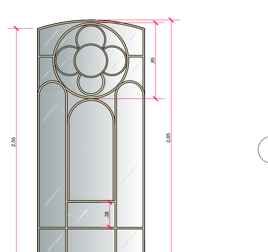
VISTA FRONTAL: JANELA 03 - VIDRO LISO / MADEIRA Escala 1:25
