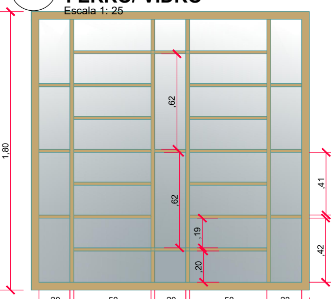
VISTA FROTAL: JANELA 11 - fixa/ basculante - MADEIRA/ VIDRO Escala 1: 25
