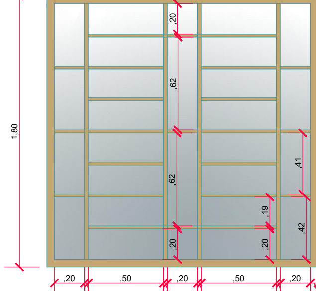
VISTA FRONTAL: JANELA 09 - fixa/ basculante - FERRO/ VIDRO Escala 1: 25
