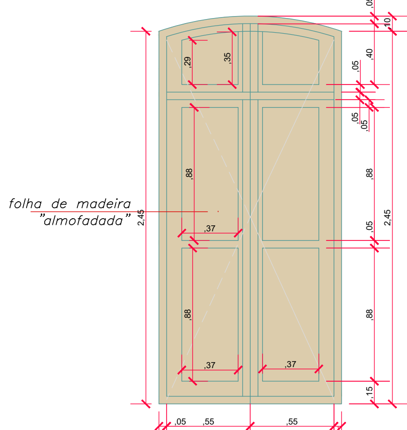
VISTA FRONTAL: JANELA 02 - ABRIR PAINEL (MADEIRA) Escala 1: 25
