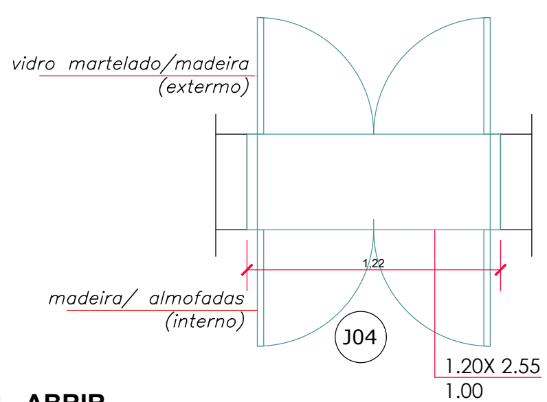
PLANTA-BAIXA: JANELA 04 - ABRIR PAINEL (MADEIRA)/ VIDRO MARTELADO Escala 1: 25
