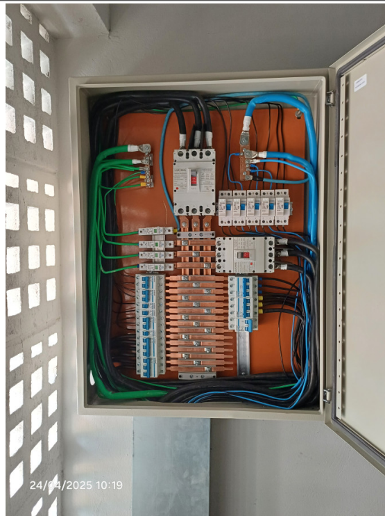
Instalação e montagem dos quadros de elétrica.
