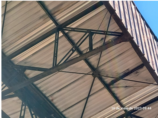
Elemento metálico em processo avançado de corrosão com necessidade de substituição.
