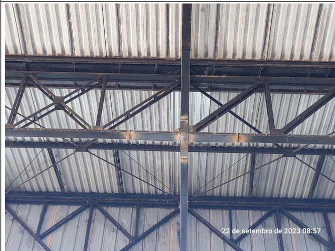
Recuperação de trecho da estrutura metálica.
