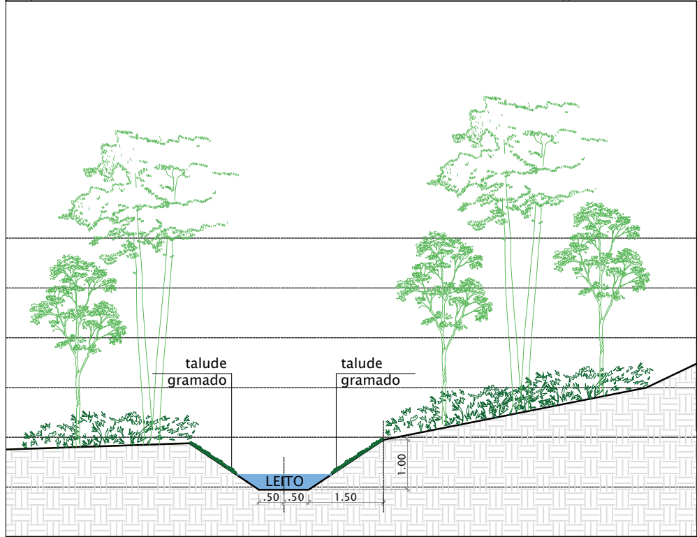
CORTE ESQUEMÁTICO ABERTURA DA VALA ESCALA 1:75
